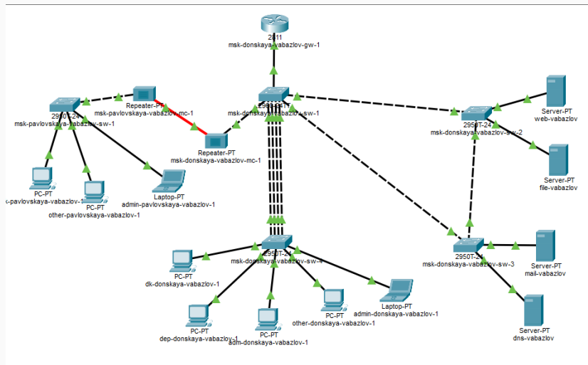
Рис. 1: Общая схема сети
