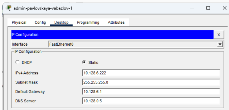
Рис. 3: Настройка второго администратора
