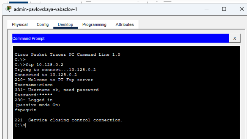
Рис. 8: Проверка FTP с другого узла
