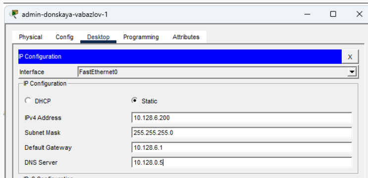
Рис. 2: Настройка IP администратора
