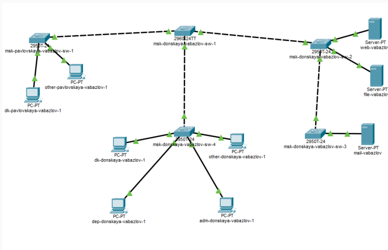
Рис. 1: Топология сети L1
