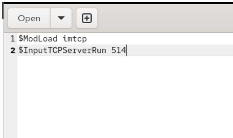
Рис. 1: Настройка netlog-server.conf
