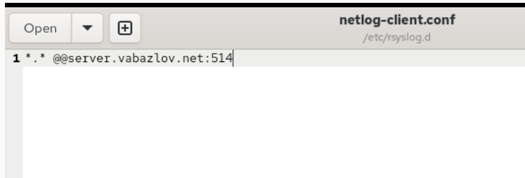
Рис. 3: Конфигурация netlog-client.conf
