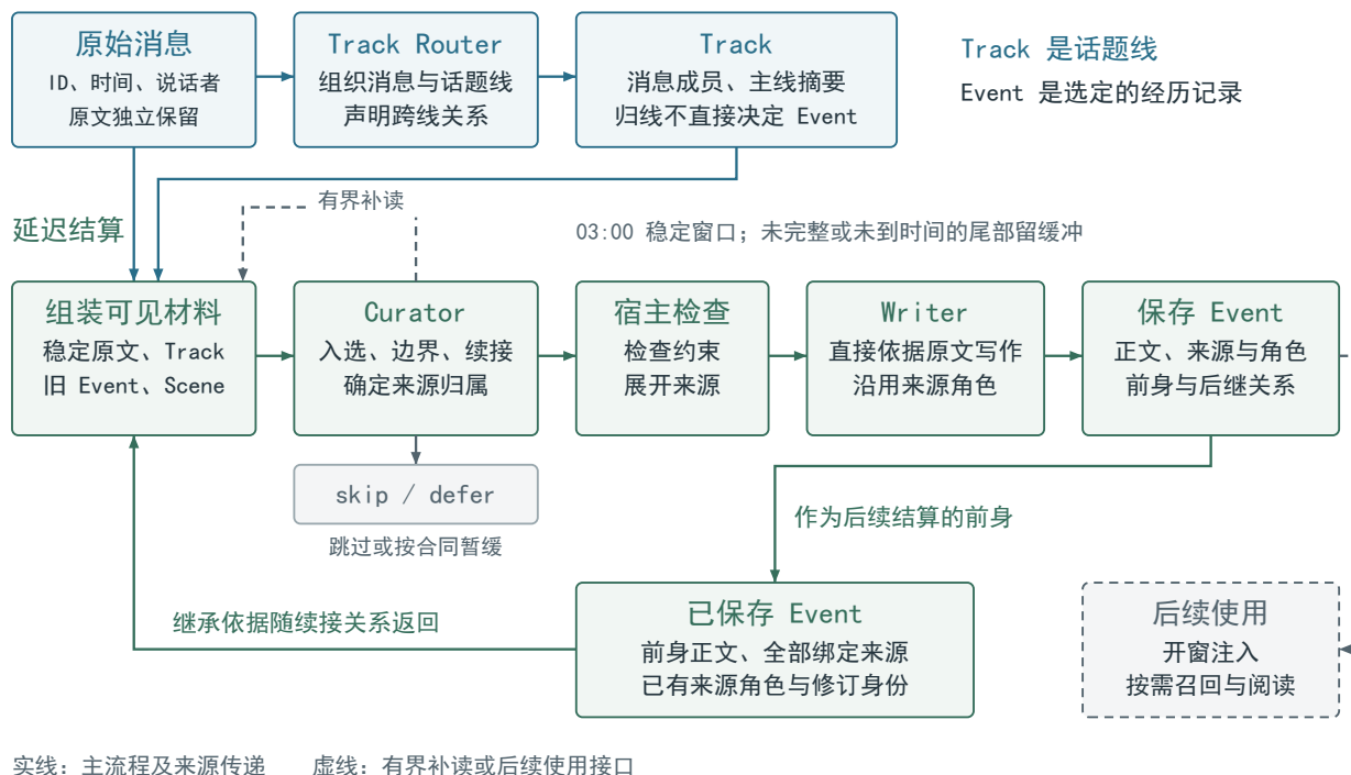
图 1. 持续归线、延迟结算与来源追溯。Track 组织话题，Curator 决定 Event 入选及续接，Writer 依据已定来源写作。补读受有界范围约束；已保存 Event 可在后续结算中作为前身。开窗注入和召回作为后续用途列于末端。图示对应 2026-09-13 核对的共同处理职责，不表示所有部署使用同一结算端点；Curator 与 Writer 之间不再调用独立证据整理模型。具体修订与部署差异见 § 3.8，各次历史执行版本见 § 4。
