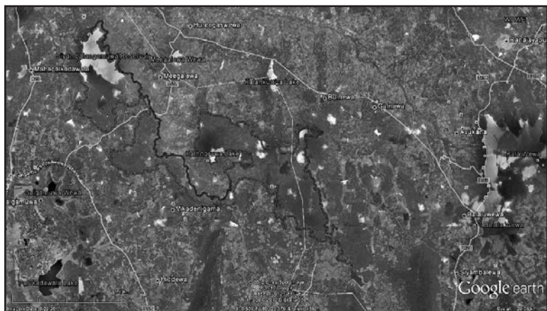
කහල්ල පල්ලේකැලේ අභයභූමියේ මායිම් දැක්වෙන චන්ද්‍රිකා ජායාරූපයක්
