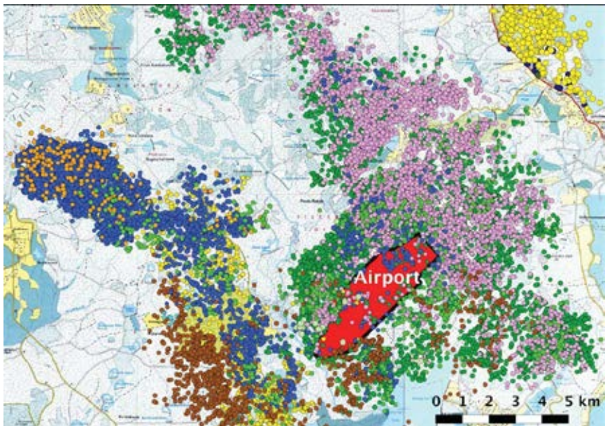
පාඨාරූපය 3.4 හම්බන්තොට දිස්ත්‍රික්කය ආශ්‍රිතව අලි ඇතුන්ගේ ව්‍යාප්තිය දැක්වෙන චන්ද්‍රිකා සිතියමක්. මෙහි මත්තල අන්තර්ජාතික ගුවන් තොටුපොළ ද දක්වා ඇත.(CCR)
