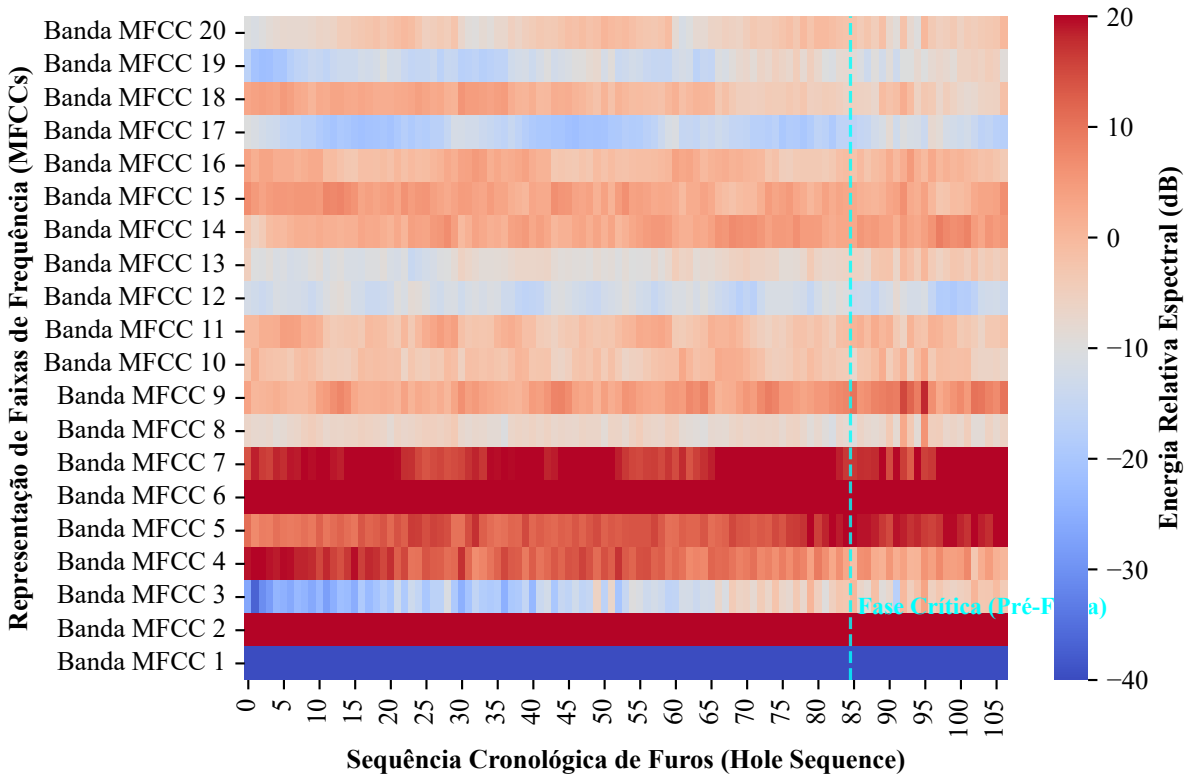
Mapeamento de Energia por Faixa de Frequência e Vida da Ferramenta (drill_4mm_05_batch_00_collet_1_30-01-2025)
