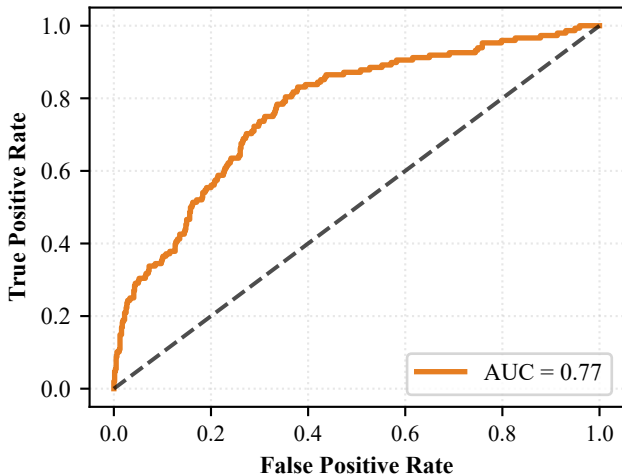
ROC Curve - XGBoost Híbrido
