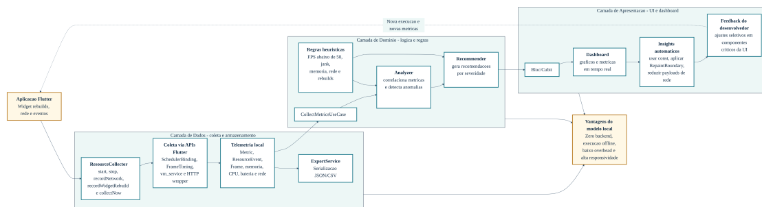
Figura 3.3: Arquitetura local e fluxo de dados do protótipo collector_flutter : coleta, análise, recomendação e apresentação no painel integrado.
