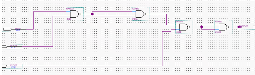
Figura 2. NAND3
