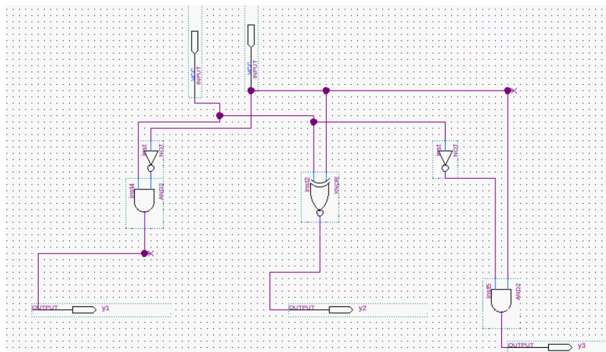
Figura 5. Comparador de 2 Bits
