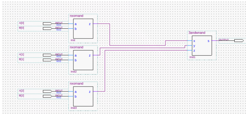
Figura 3. Circuito Completo
