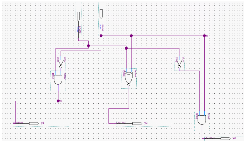
Figura 4. Comparador de 1 Bit
