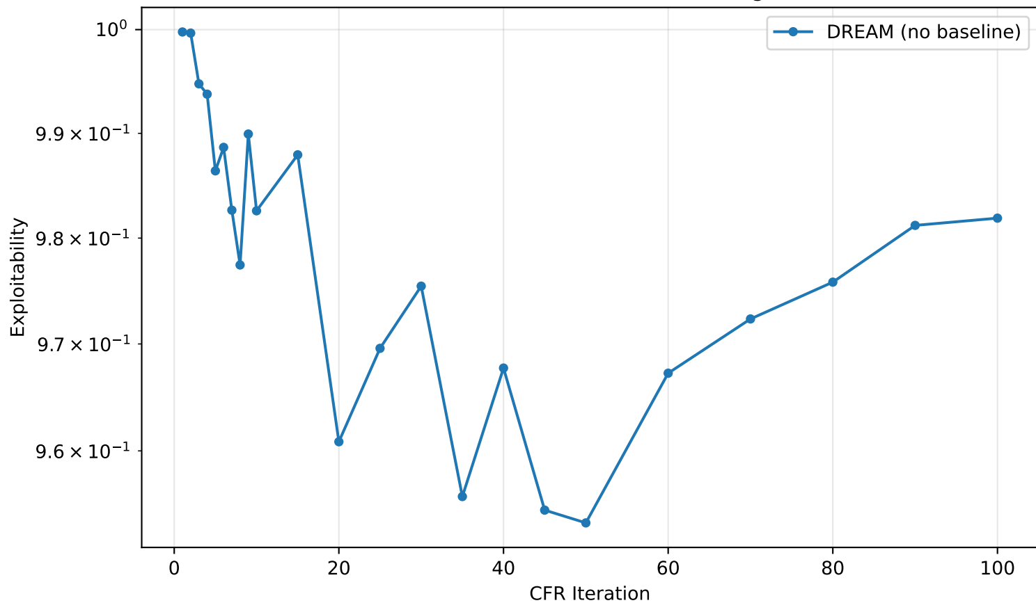
3x3 CDH Dark Hex: DREAM Convergence
