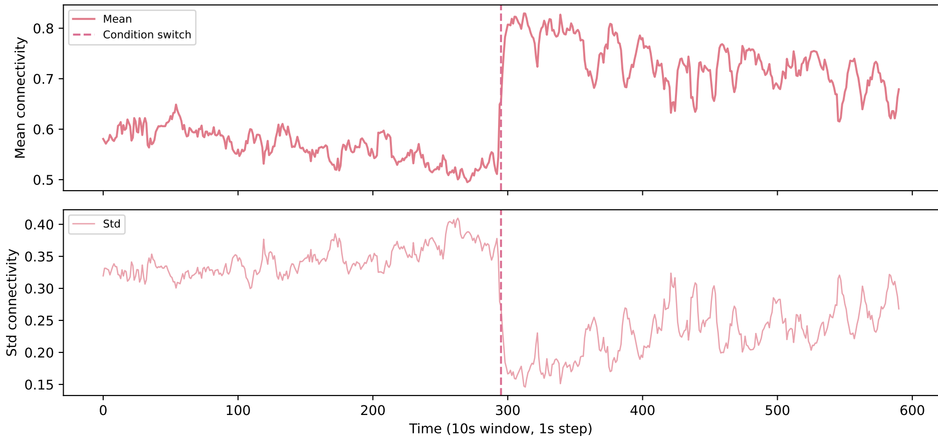
C01 — Frontal &lt;-&gt; Frontal
