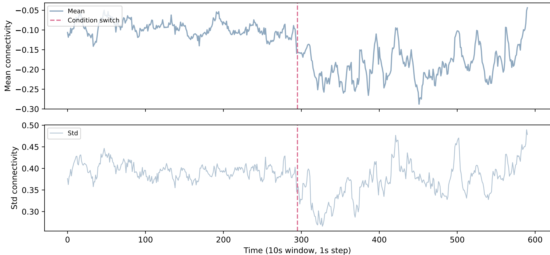
C01 — Parietal <-> Reference
