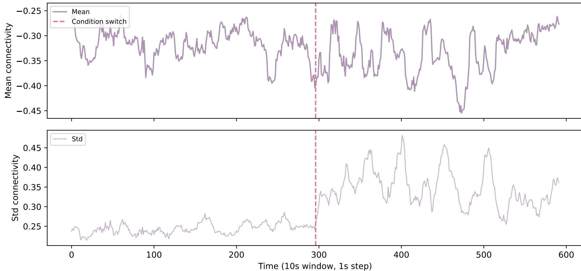
C03 — Frontal &lt;-&gt; Parietal
