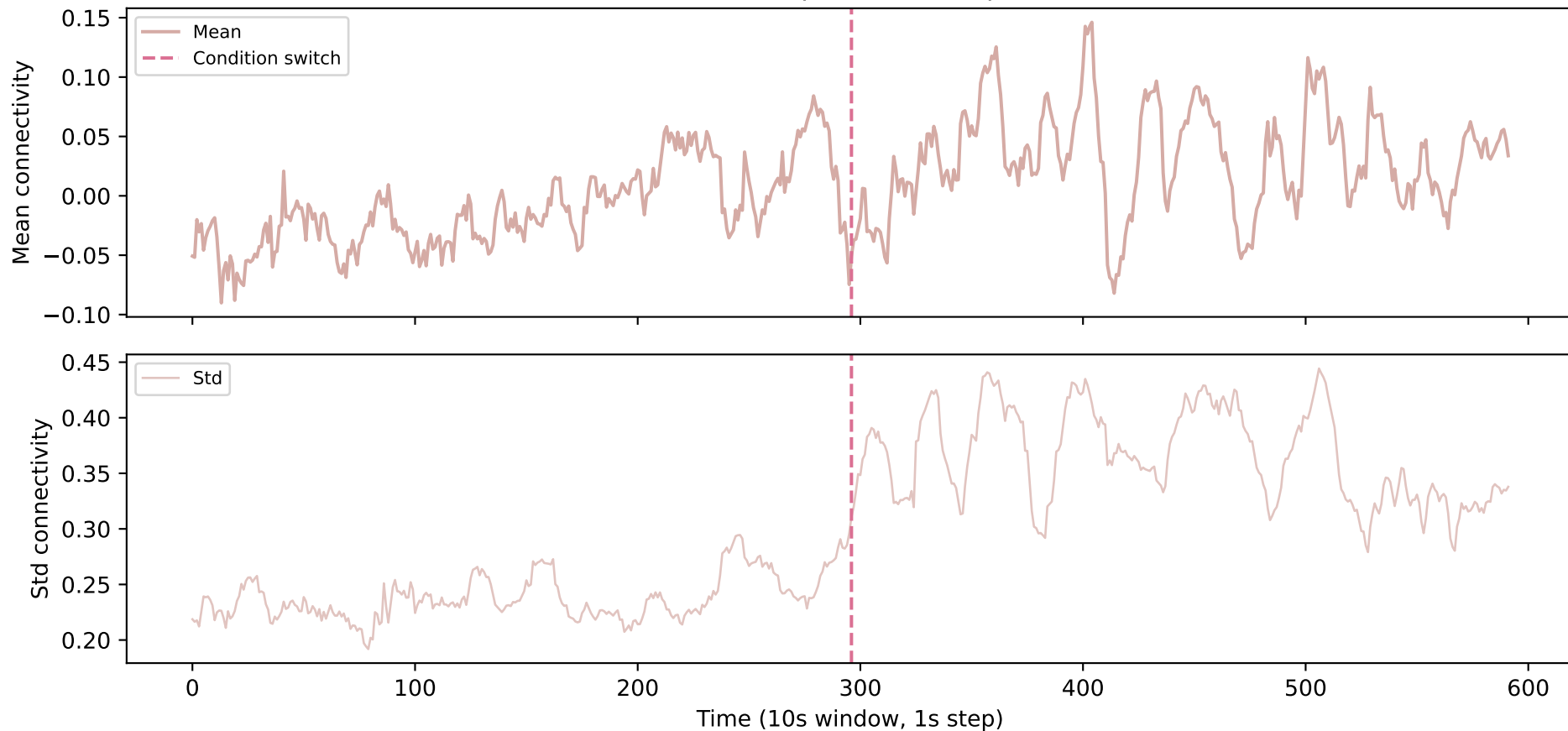
C03 — Occipital <-> Temporal
