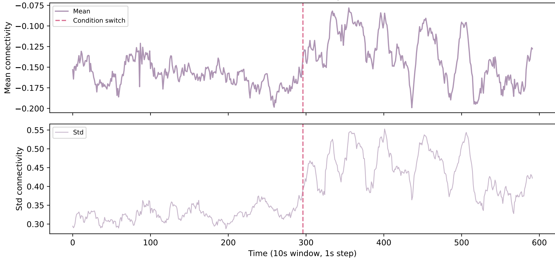
C03 — left &lt;-&gt; right
