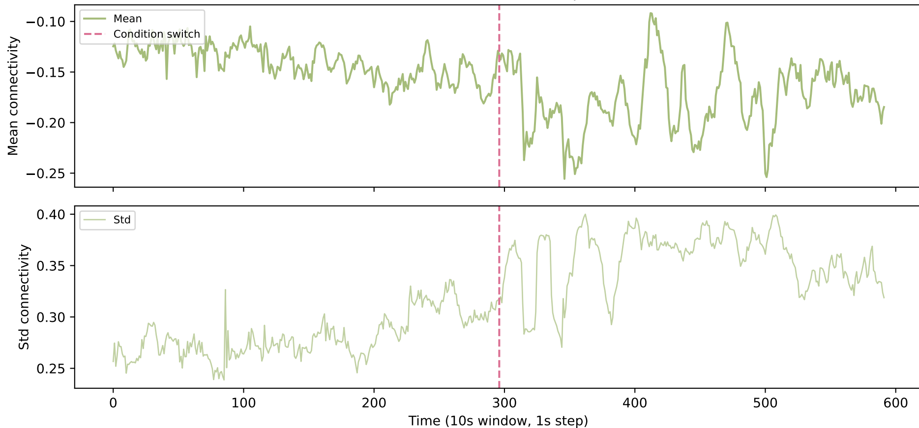
C03 — Central \leftrightarrow Temporal
