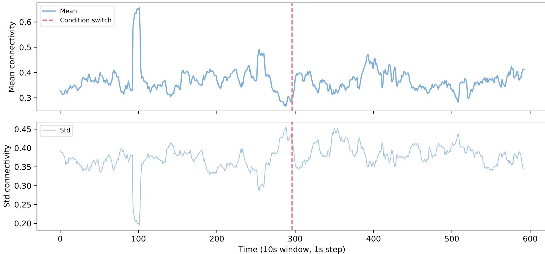
C05 — Parietal <-> Parietal
