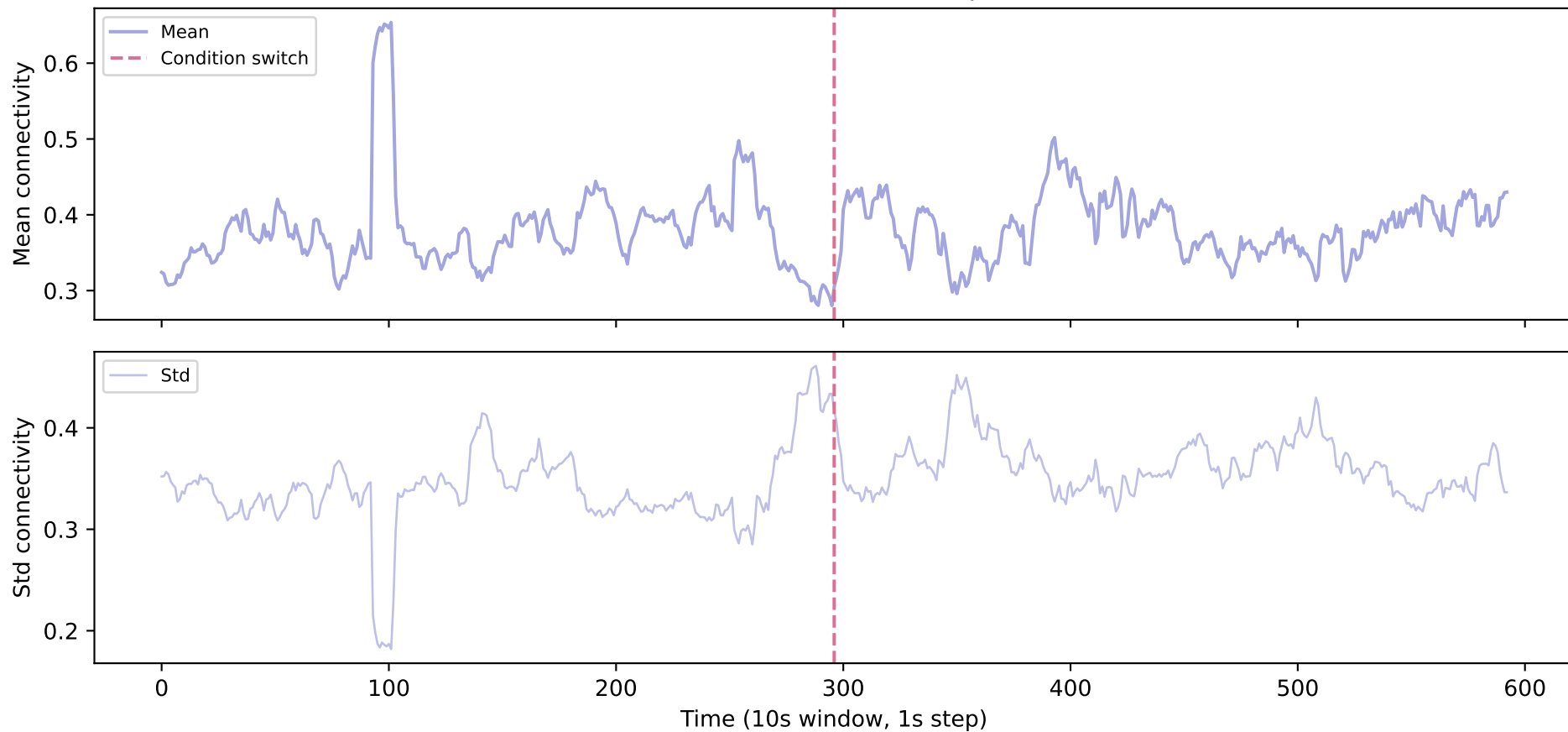
C05 — Parietal <-> Occipital
