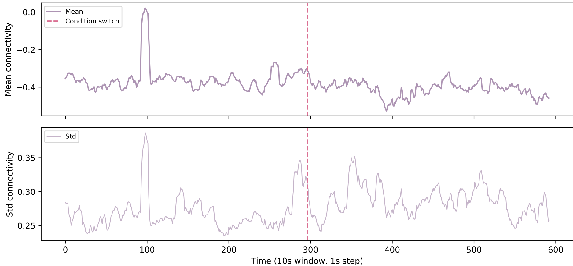
C05 — Frontal <-> Parietal
