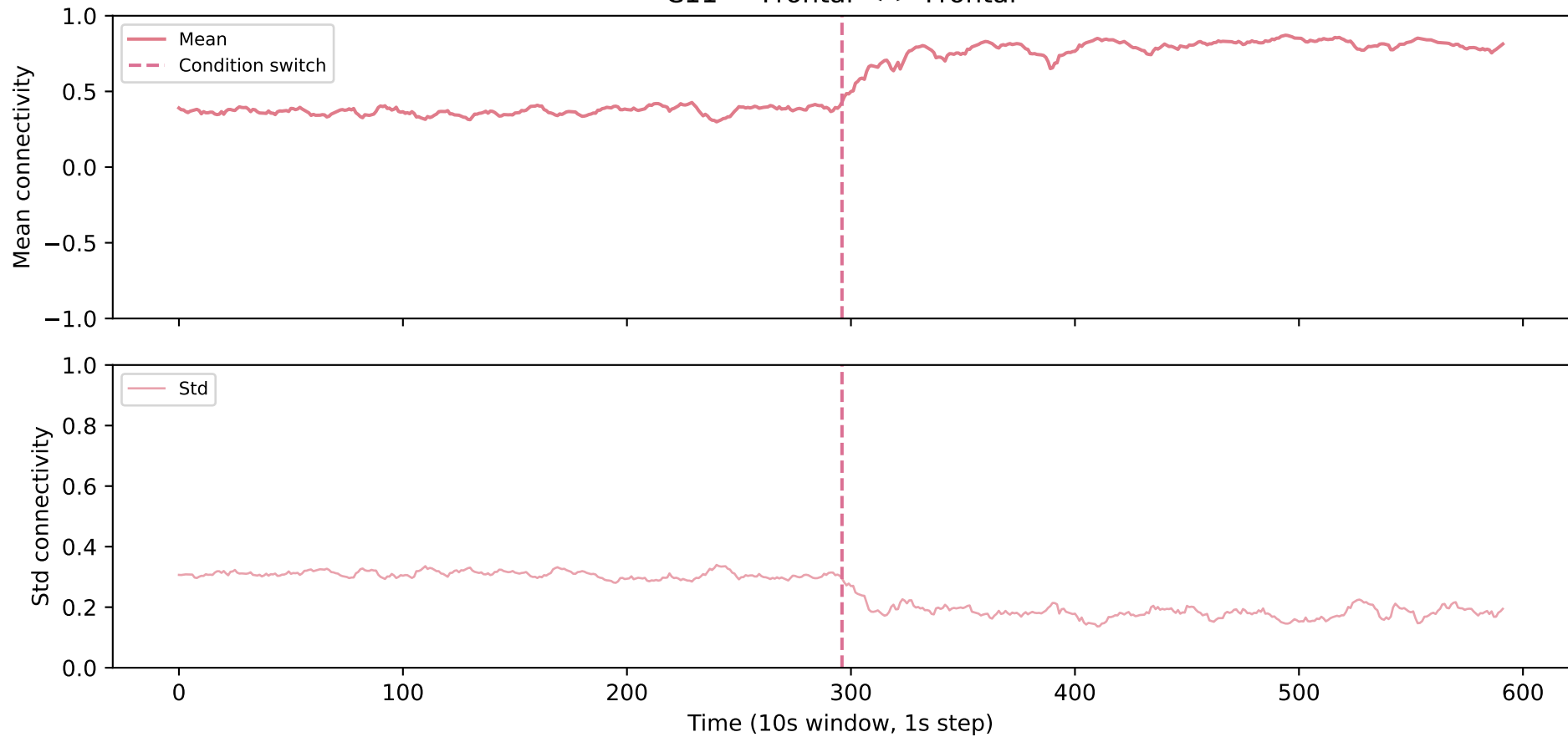
C11 — Frontal &lt;-&gt; Frontal
