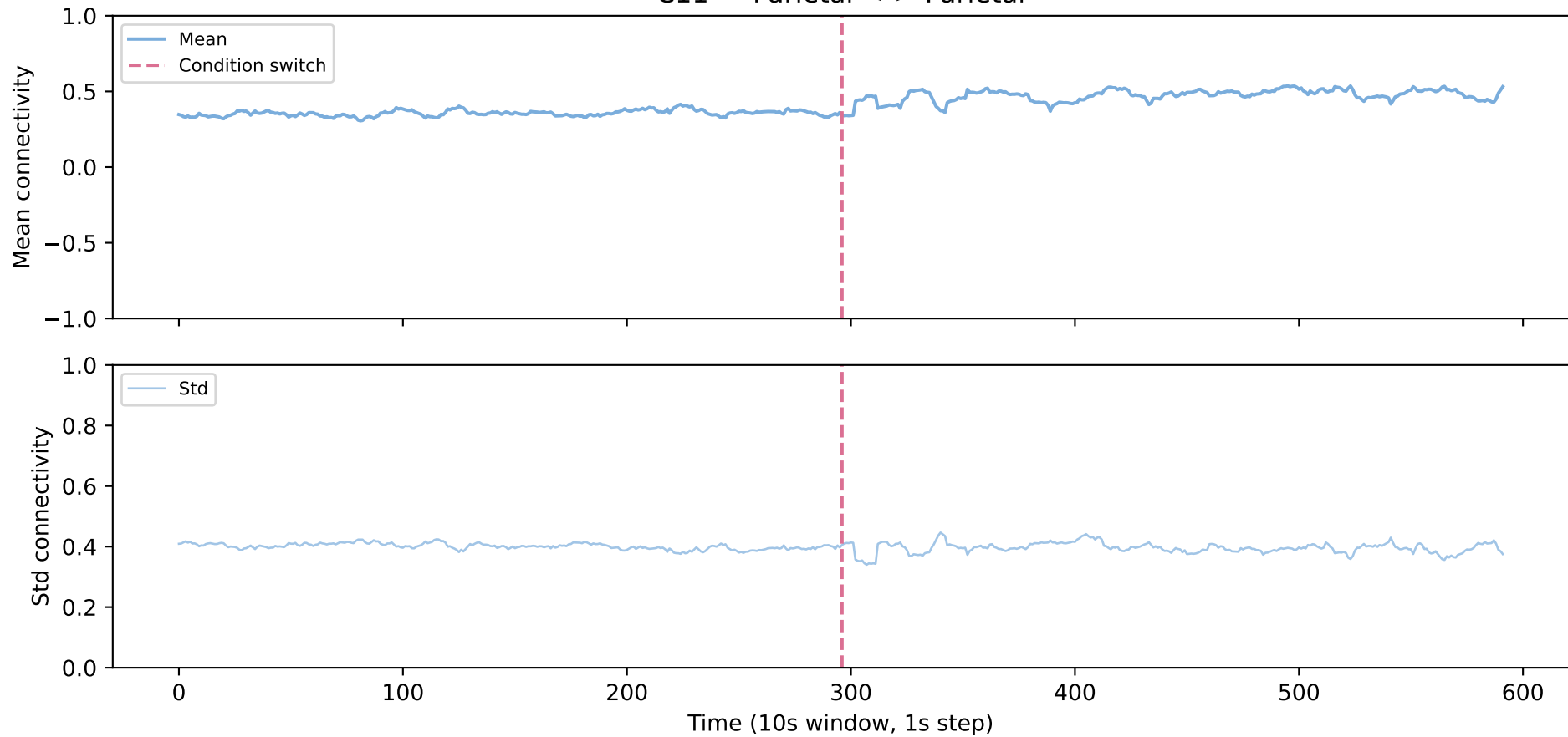
C11 — Parietal &lt;-&gt; Parietal
