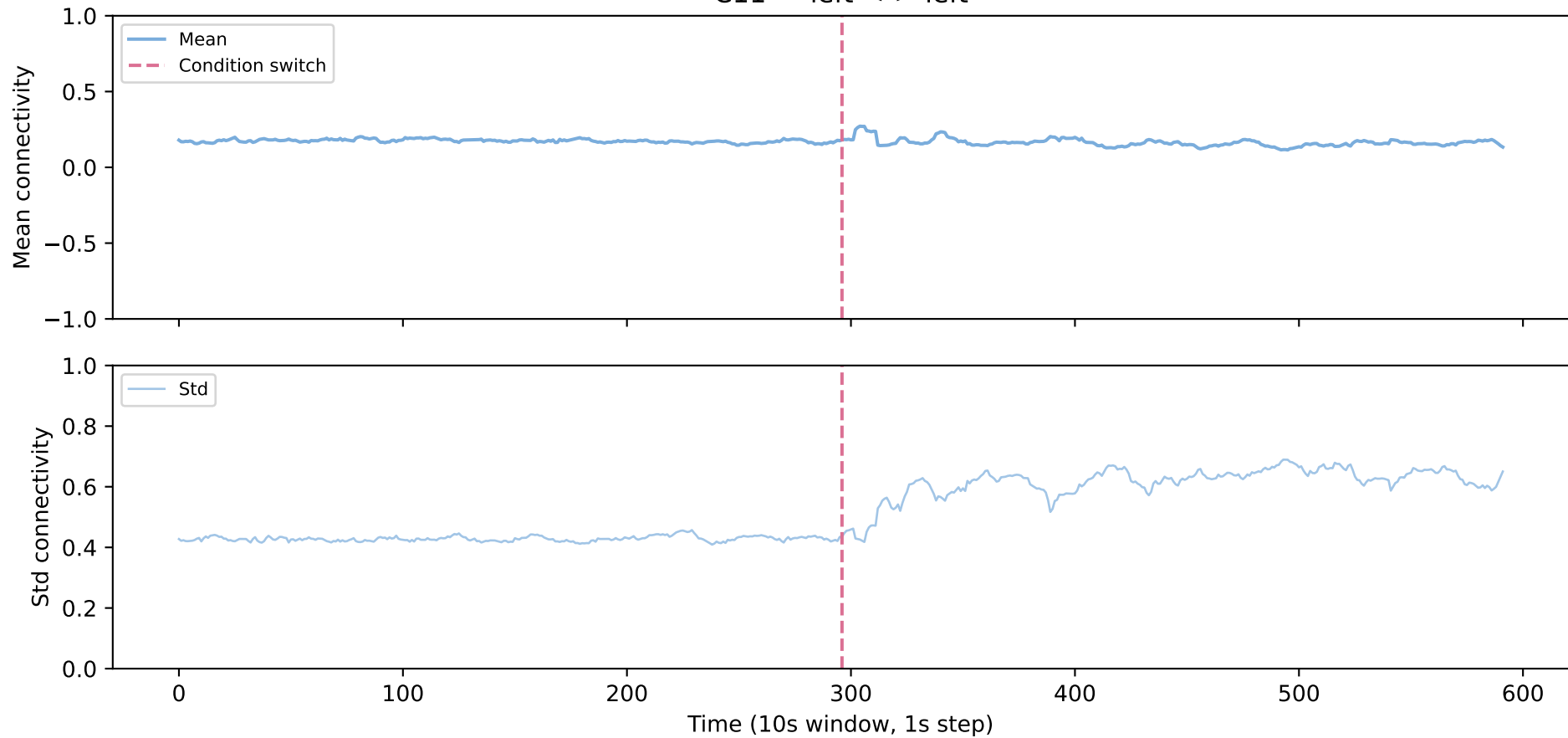
C11 — left <-> left
