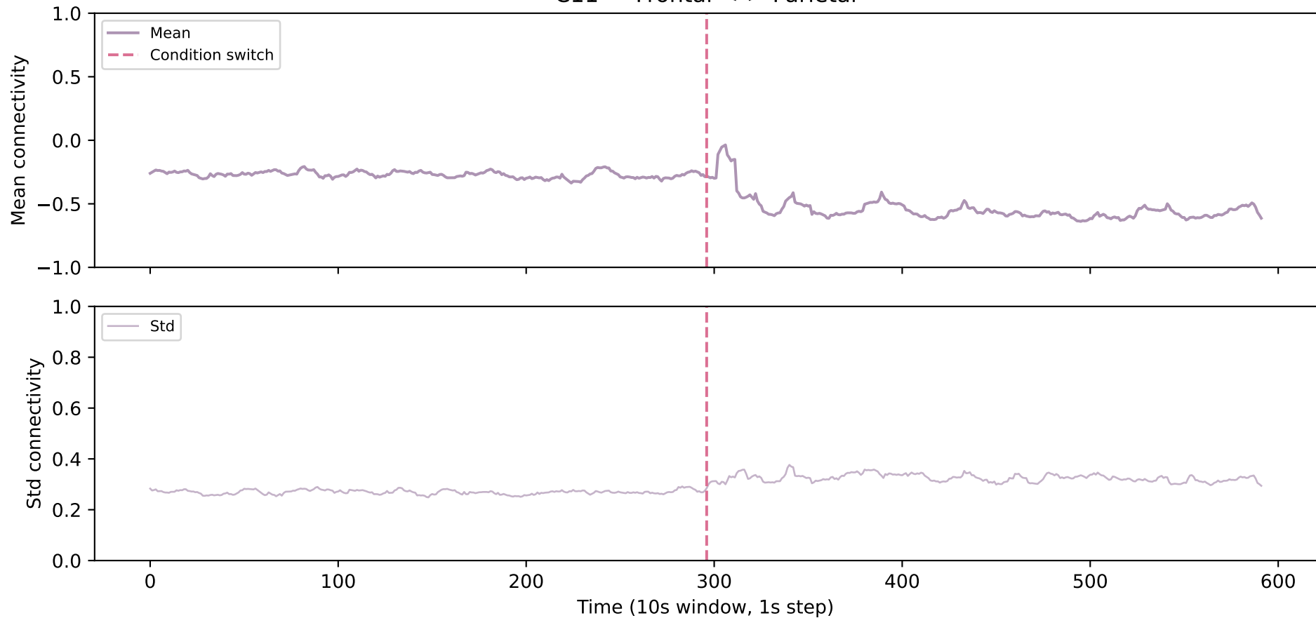
C11 — Frontal &lt;-&gt; Parietal
