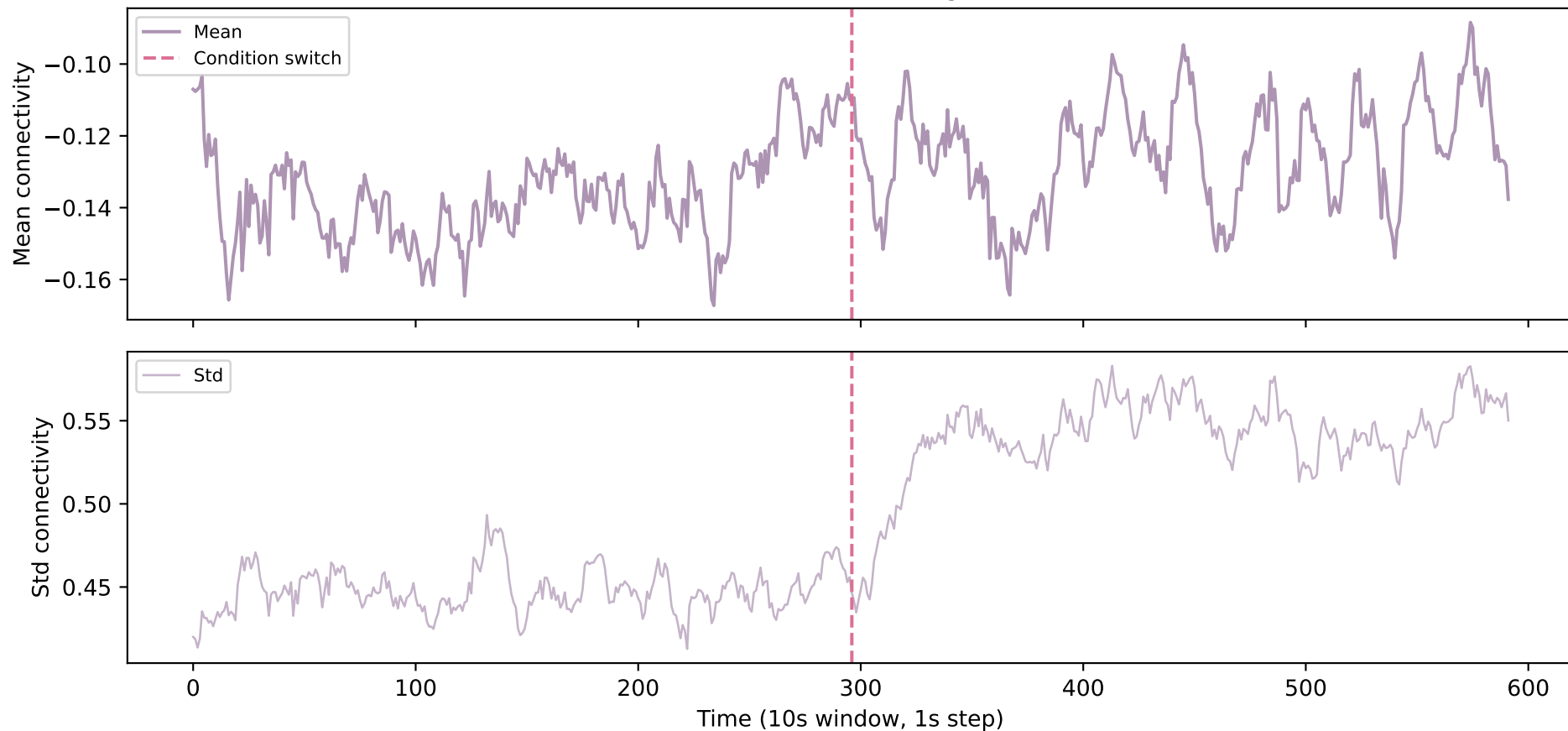
C15 — left <-> right
