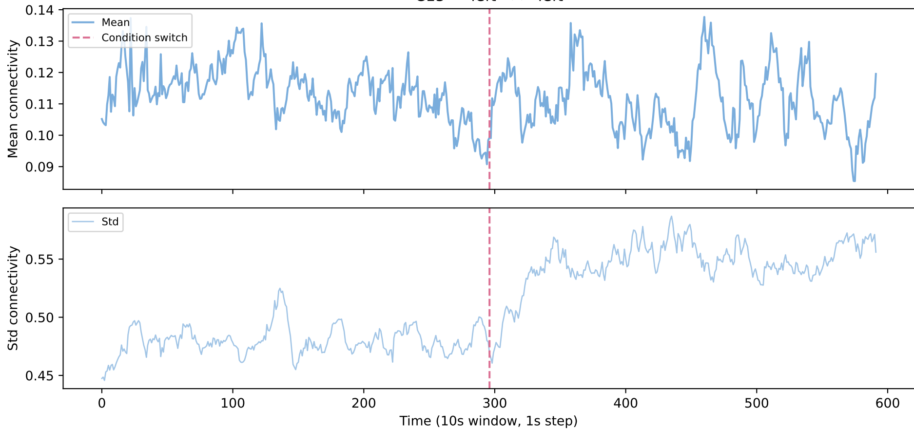
C15 — left <-> left
