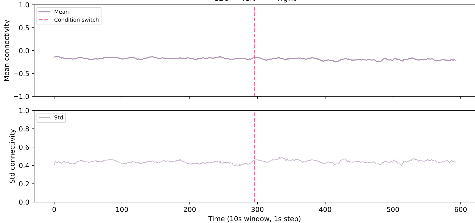
C20 — left <-> right
