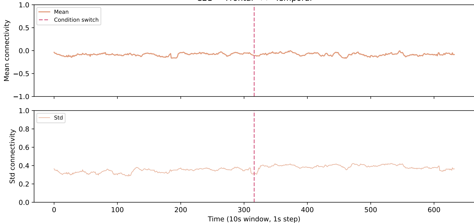
C21 — Frontal <-> Temporal
