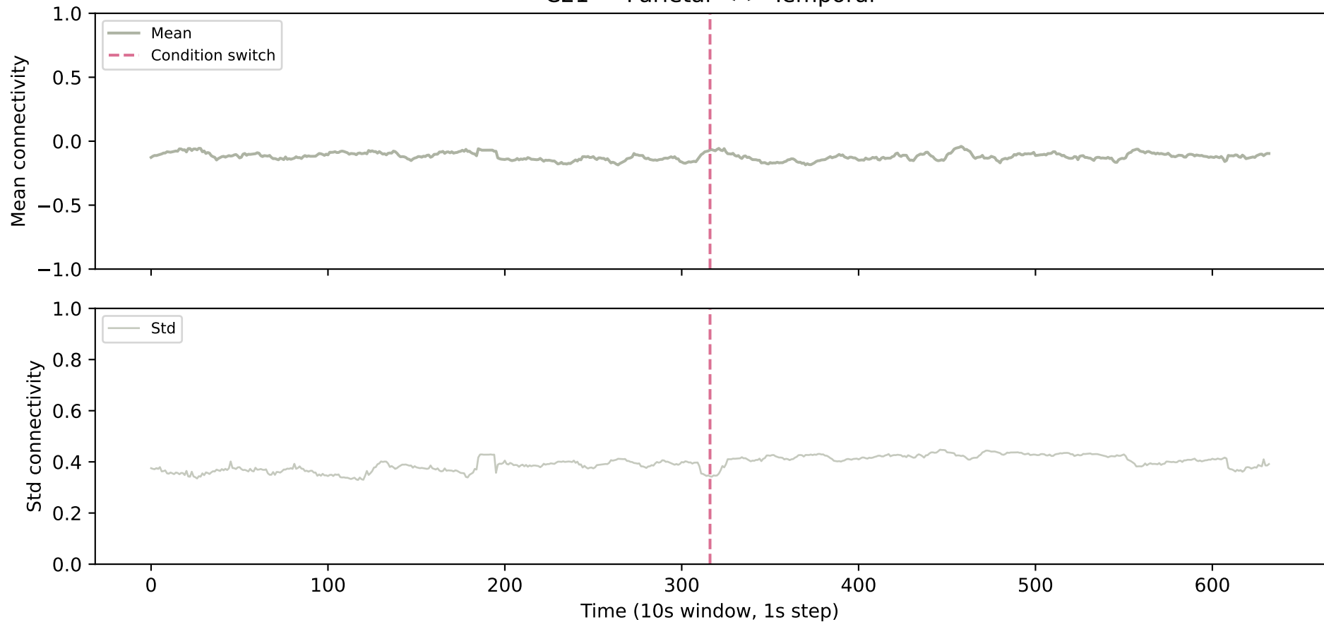
C21 — Parietal <-> Temporal
