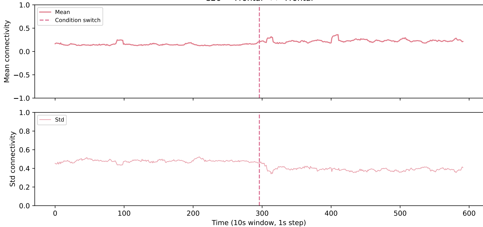
C26 — Frontal &lt;-&gt; Frontal
