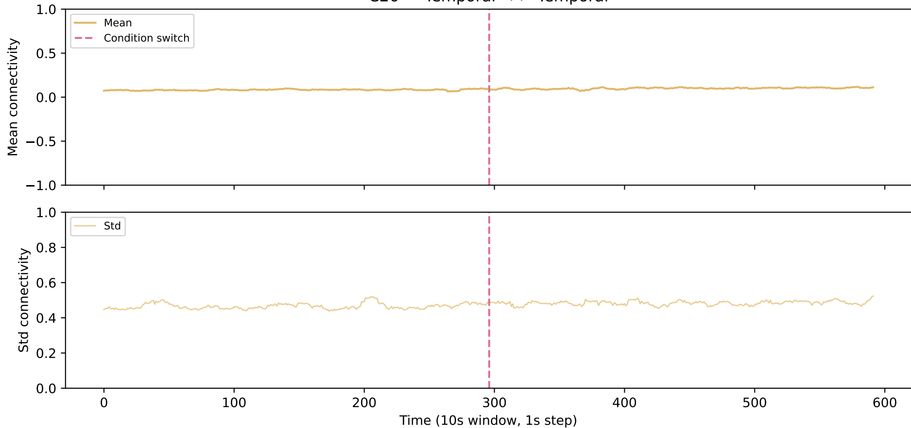
C26 — Temporal \leftrightarrow Temporal
