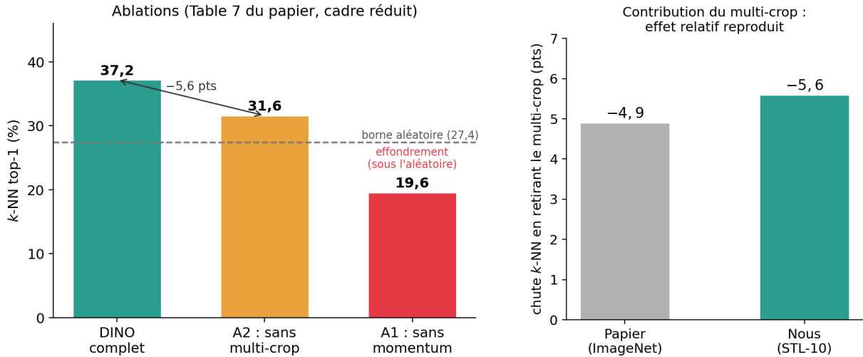
FIGURE 4 – Gauche : ablations en cadre réduit. Retirer le momentum (A1) effondre la représentation sous la borne aléatoire ; retirer le multi-crop (A2) coûte -5,6 points. Droite : la contribution du multi-crop que nous mesurons ( -5,6 pt) coïncide presque avec celle du papier ( -4,9 pt, Table 7), bien que l’échelle diffère d’un facteur \sim 50 .
