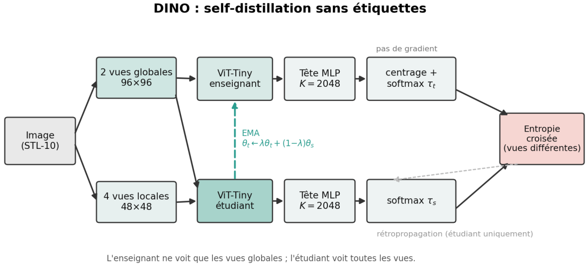
FIGURE 1 – Architecture de DINO. Une image produit 2 vues globales ( 96 \times 96 ) et 4 vues locales ( 48 \times 48 ). L’enseignant — moyenne mobile (EMA) de l’étudiant, non entraîné par rétropropagation — ne traite que les vues globales ; l’étudiant traite toutes les vues. Chaque branche enchaîne un ViT-Tiny puis une tête de projection ( K = 2048 ) ; la perte est l’entropie croisée entre la distribution enseignant (centrée puis affûtée) et la distribution étudiant , sur les paires de vues différentes.
