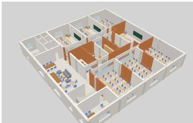
Butun qavat — tepadan umumiy ko'rinish (to'q sariq — yangi devorlar)
