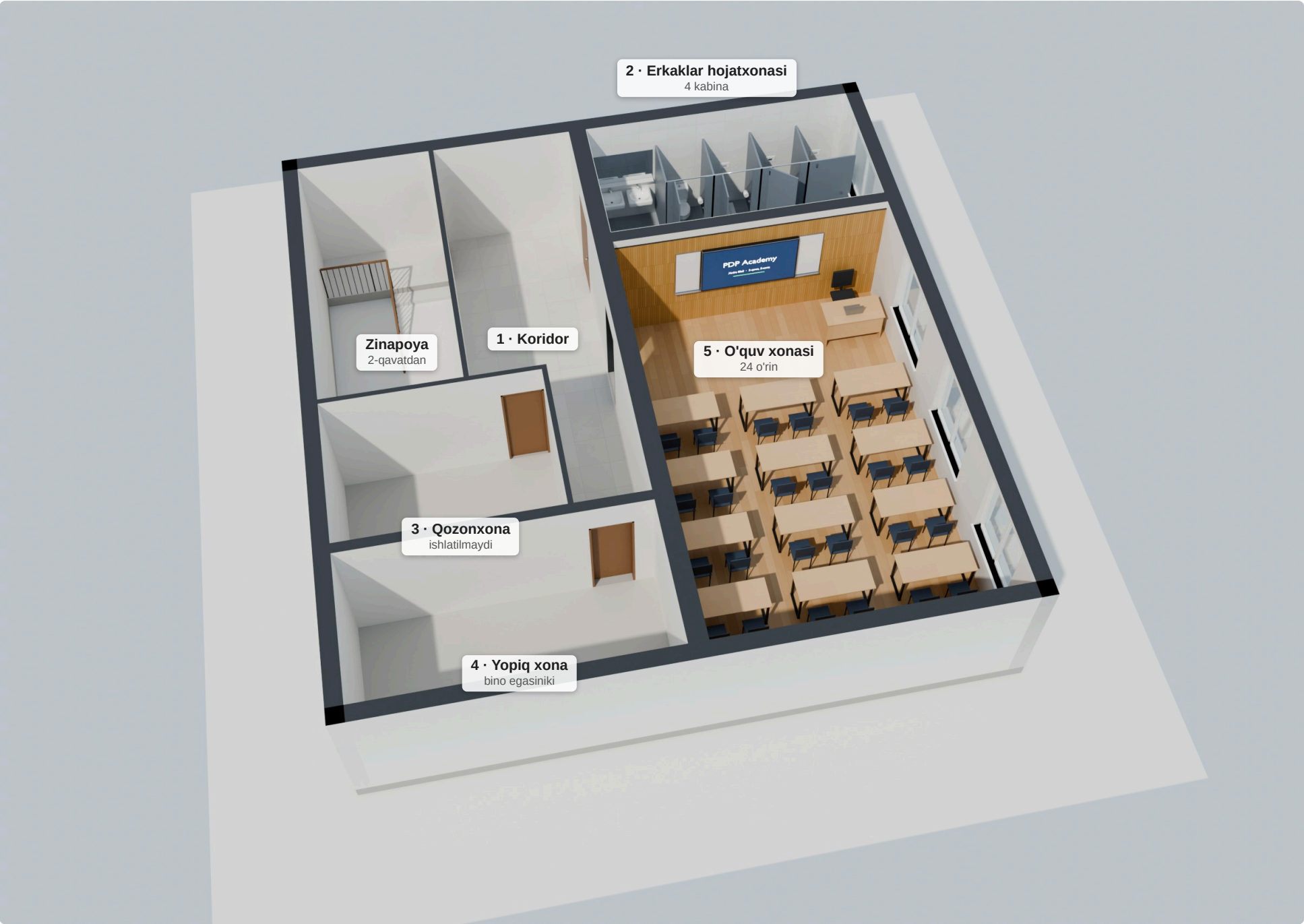
1 Umumiy ko'rinish — janubi-g'arbdan, shift olib tashlangan, devorlar 2.7 m da kesilgan. Bino 11.85 × 12.3 m, umumiy 118 m².
