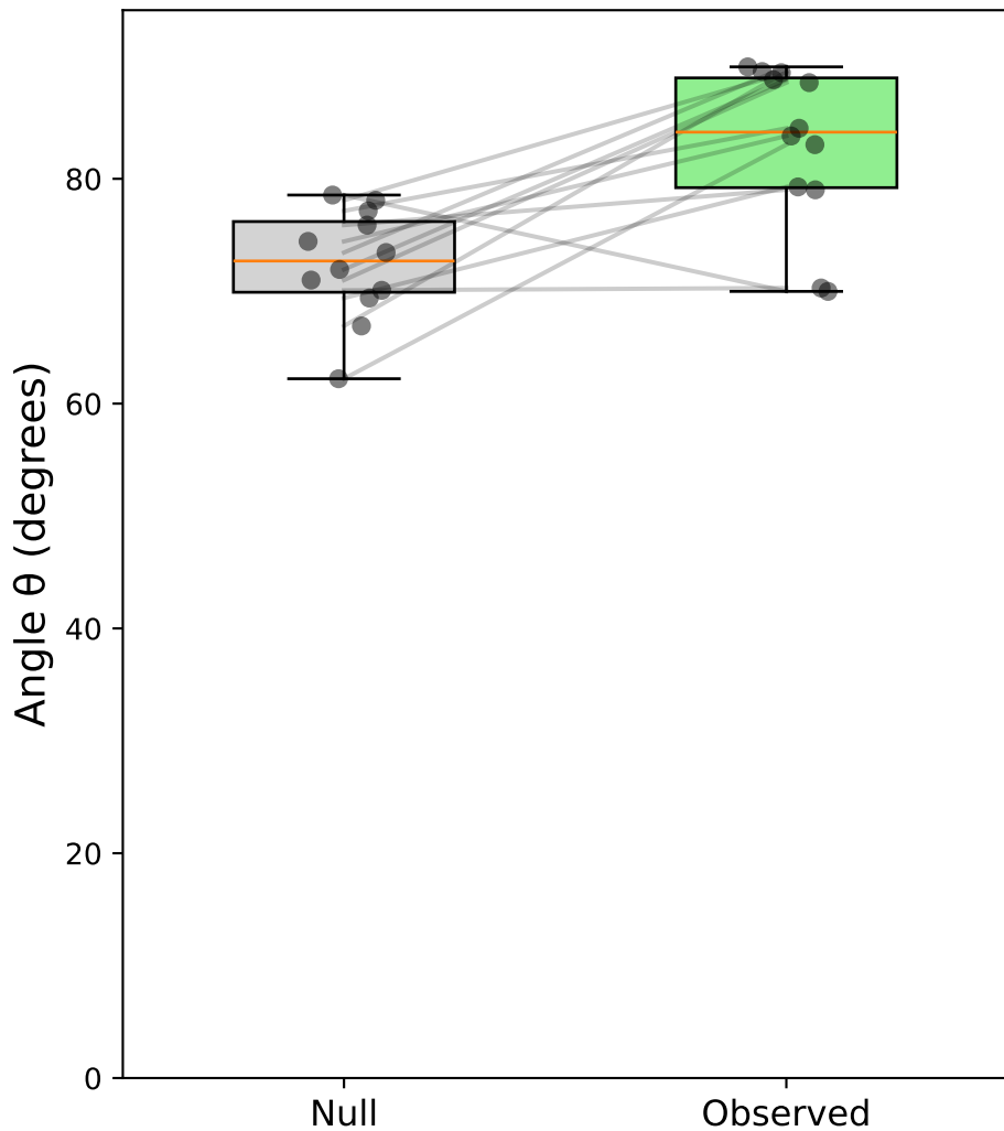
Case vi: Sacc C&S (vert, all) - Monkey S \Delta\theta = 10.6^\circ
