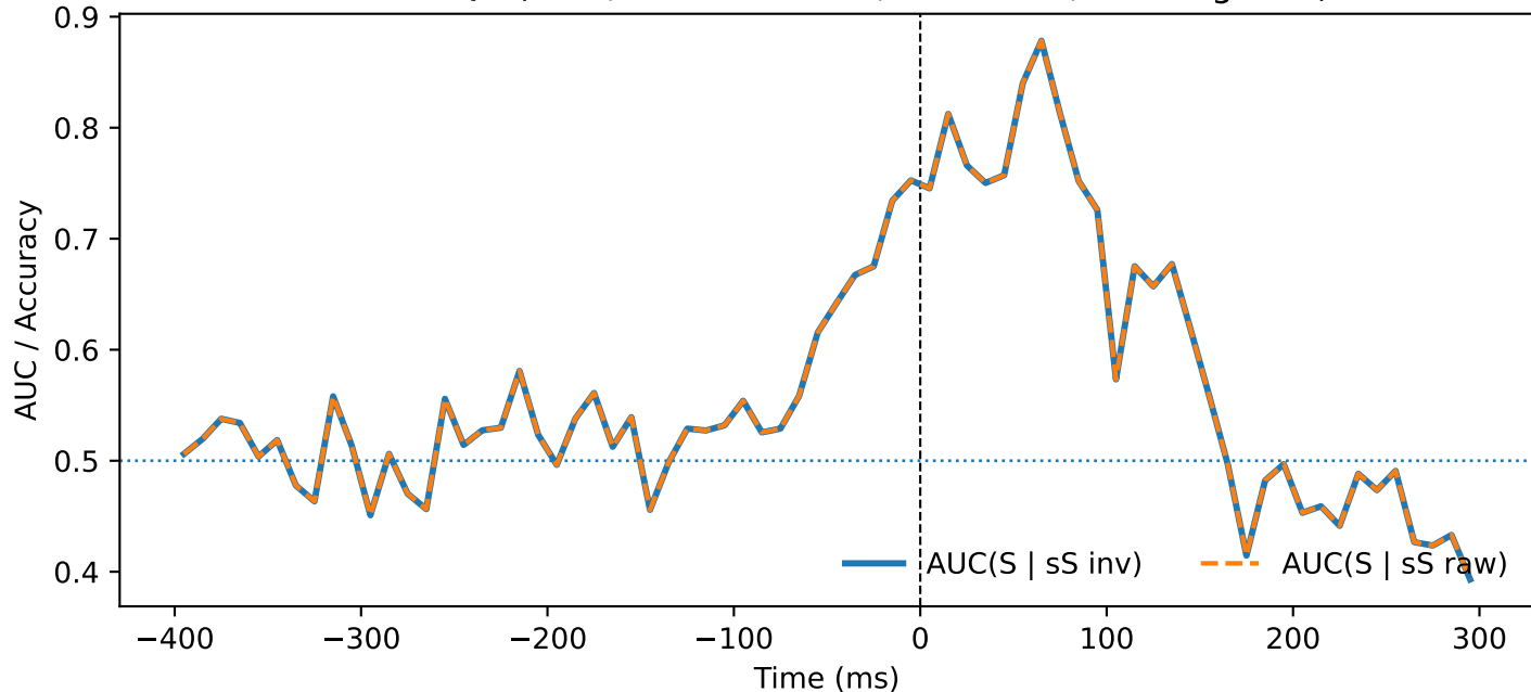
SLIP — QC (sacc, ori=horizontal, PT \geq 200.0, norm=global)
