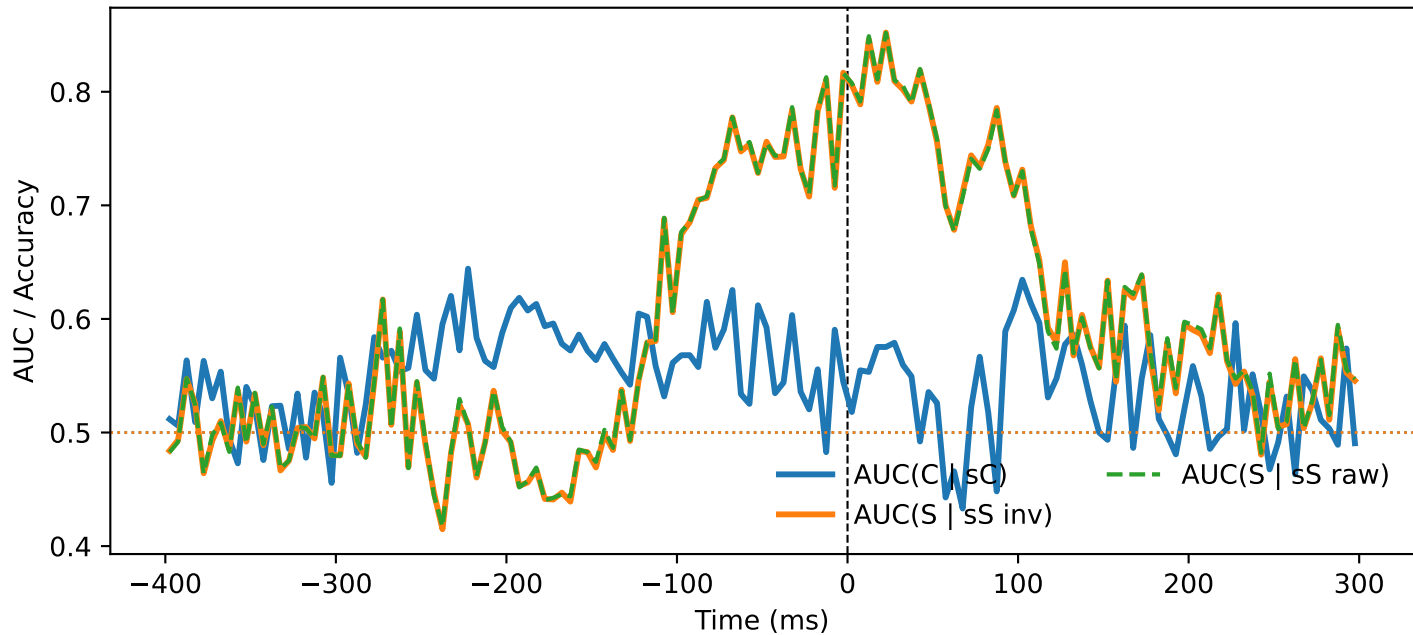
MLIP — QC (sacc, ori=horizontal, PT \geq 200.0)
