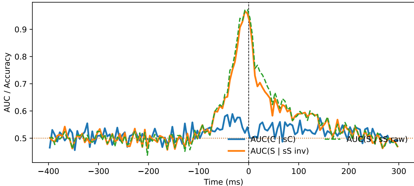
SSC — QC (sacc, ori=None, PT \geq 200.0)
