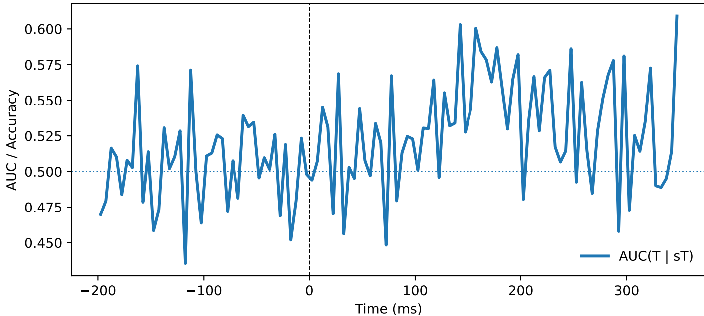
SSC — QC (targ, ori=horizontal, PT \geq 200.0)
