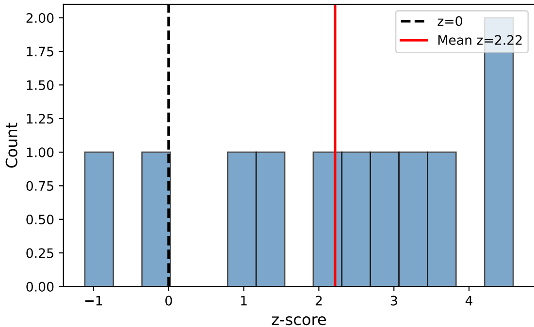
Case iii: Stim-C(vert) vs Sacc-S(horiz) (correct) - Monkey M
