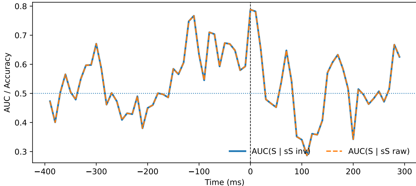
SSC — QC (sacc, ori=horizontal, PT \geq 200.0, norm=global)
