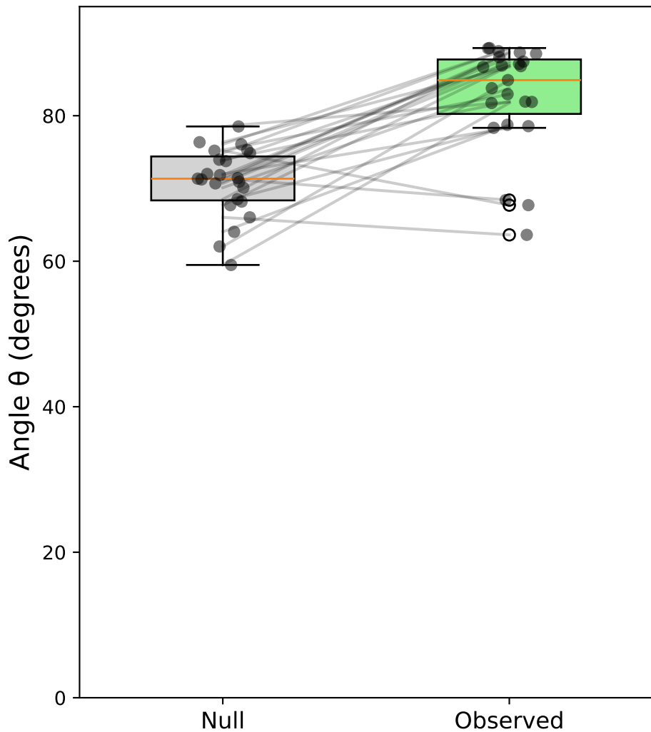
Case vi: Sacc C&S (vert, correct) - Monkey all \Delta\theta = 11.8^\circ
