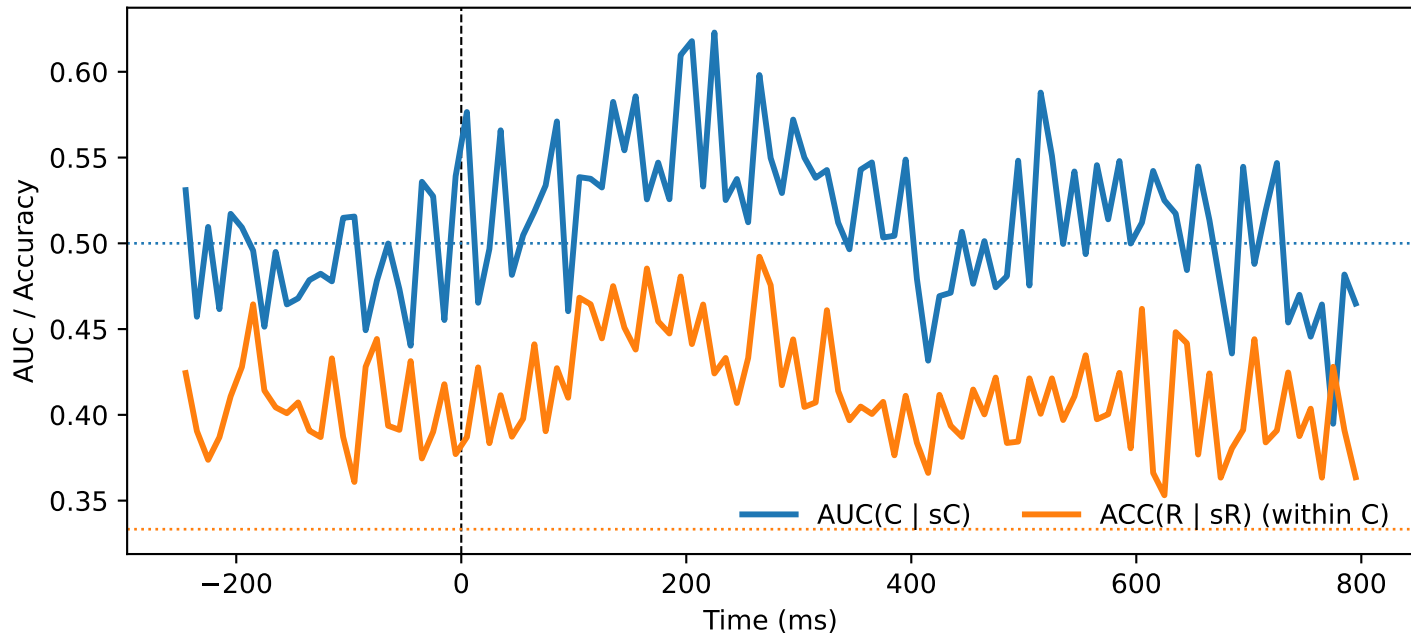
MSC — QC (stim, ori=horizontal, PT \geq 200.0)
