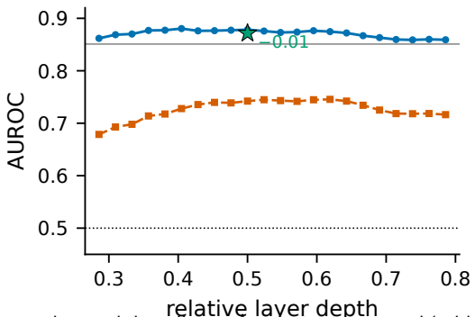
Gemma-2-9B
