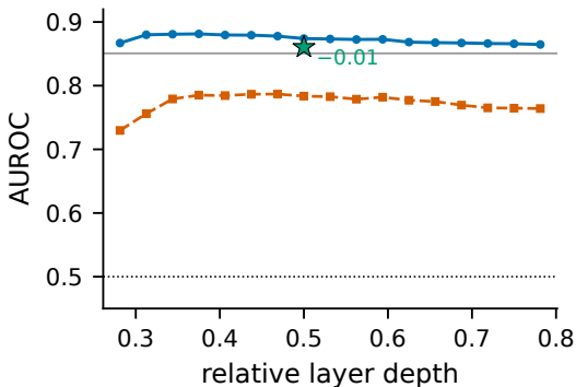
Gemma-2-9B
