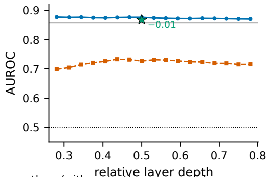
Llama-3.1-8B
