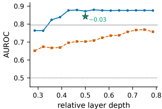
Llama-3.1-8B
