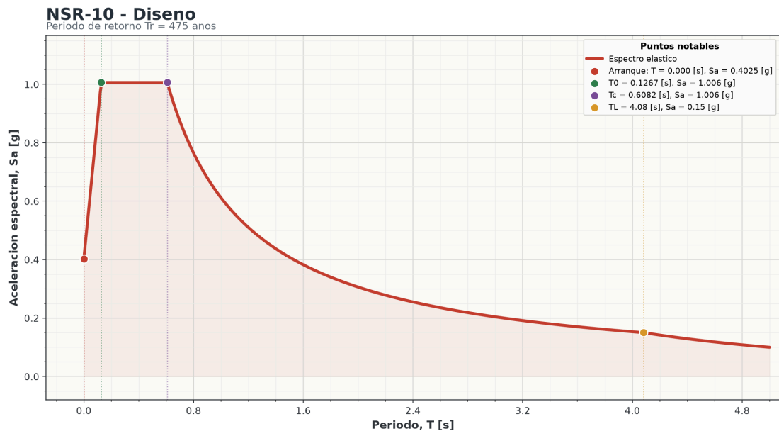
Figura 3: Espectro NSR-10 de diseño.
