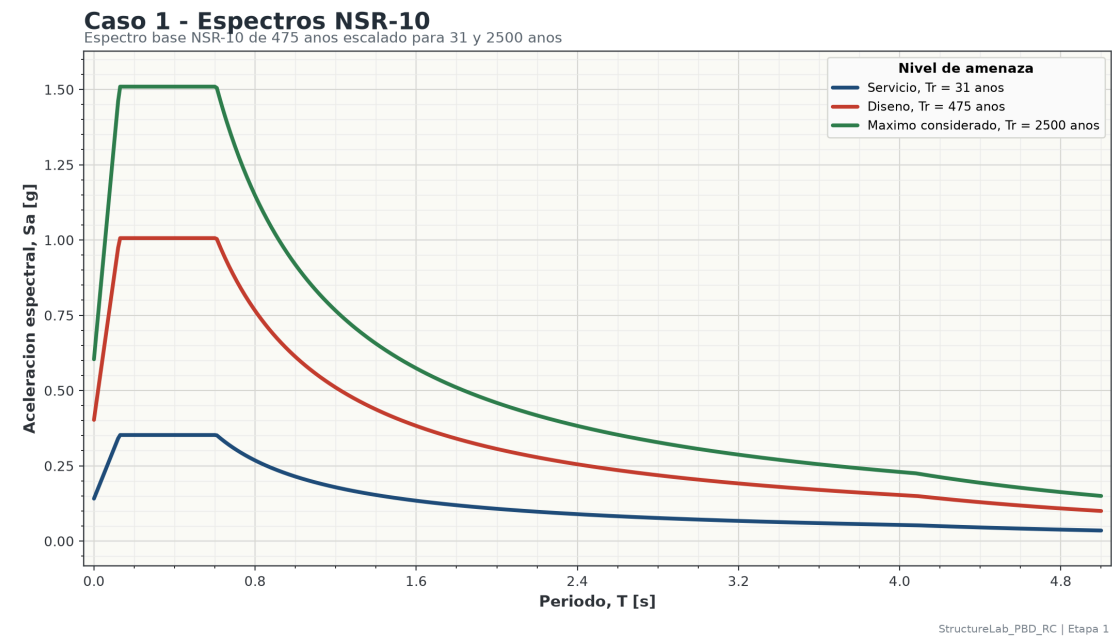
Figura 1: Espectros NSR-10 por nivel de amenaza.
