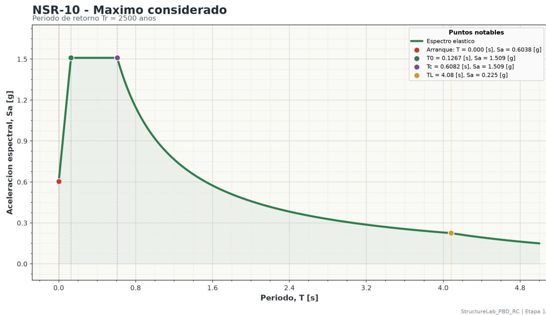
Figura 4: Espectro NSR-10 maximo considerado.
