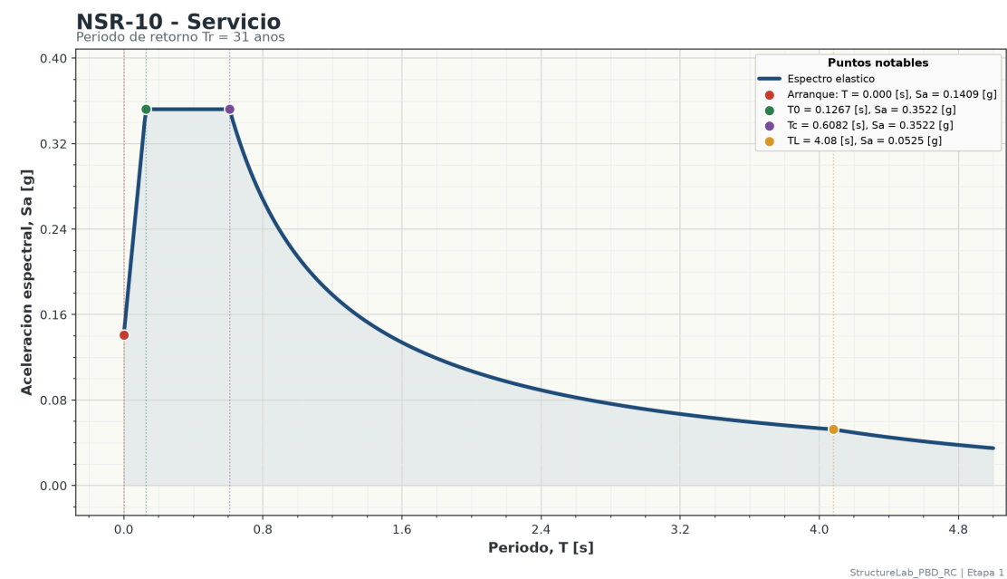
Figura 2: Espectro NSR-10 de servicio.
