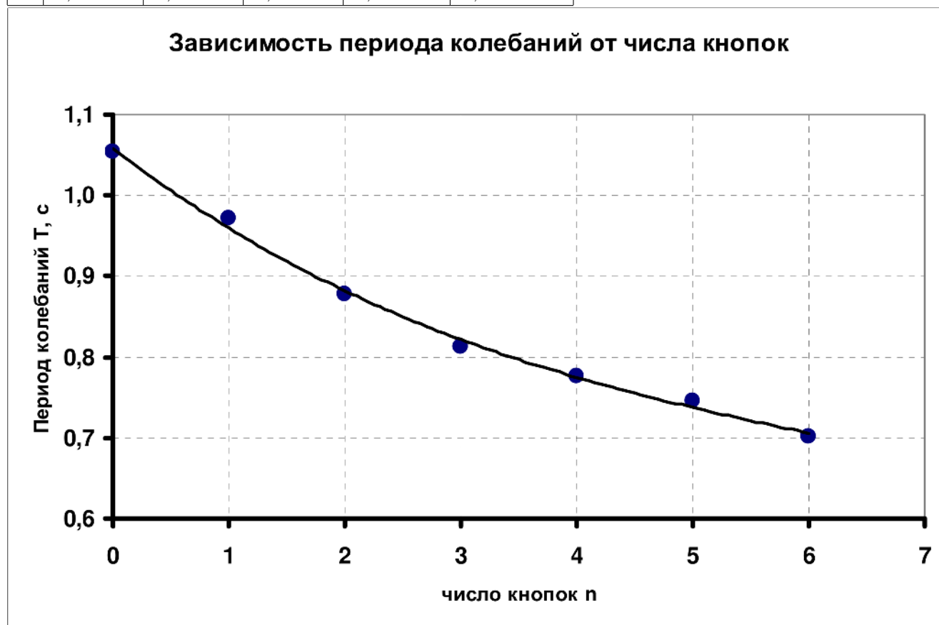
Зависимость периода колебаний от числа кнопок
