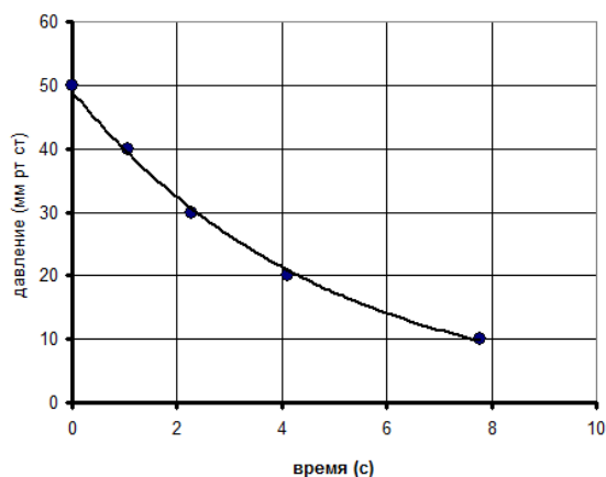
Зависимость давления от времени в воздухе
