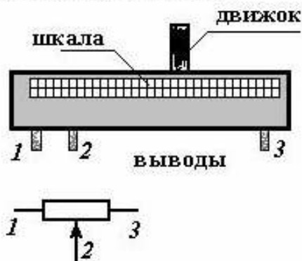
Полосковый реостат
