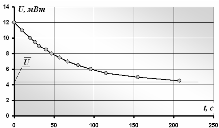
Рис. 4 Зависимость напряжения от времени
