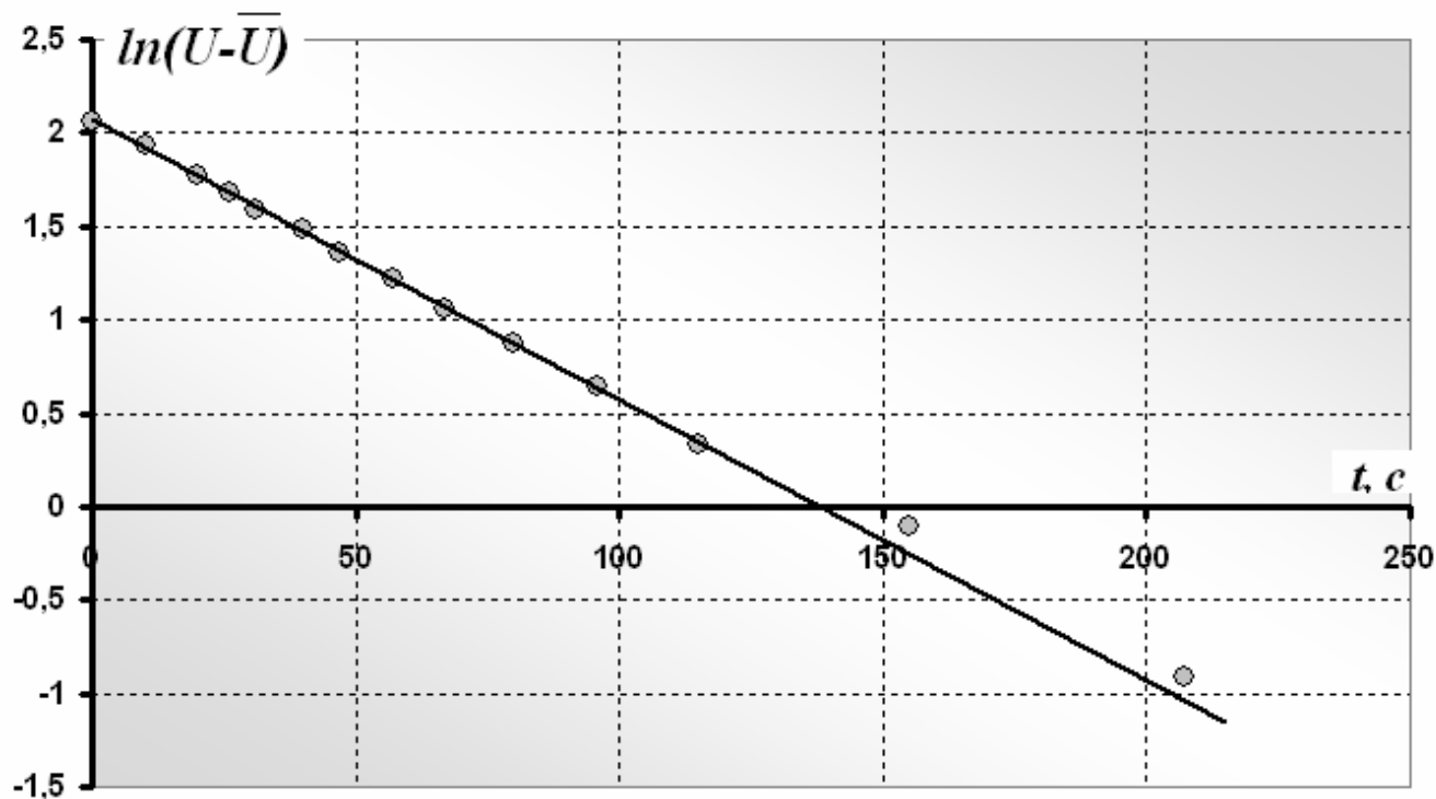
Рис. 6 Зависимость напряжения от времени (полулогарифический масштаб)
