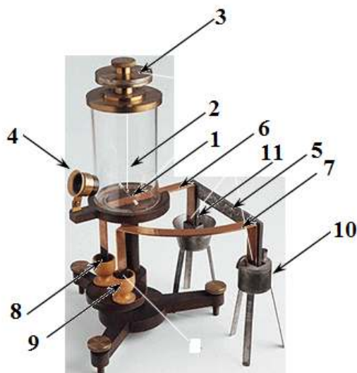
Прибор Г. Ома
