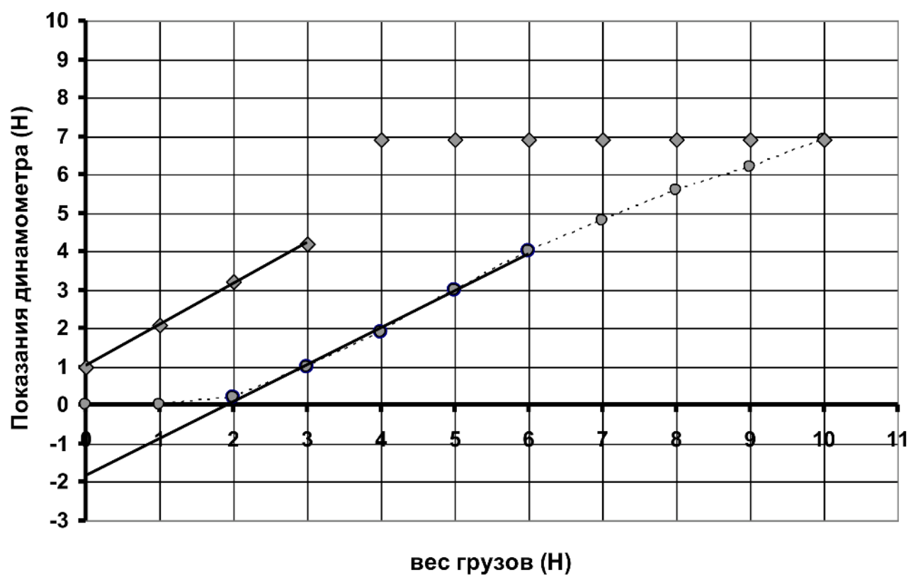
Зависимость показаний динамометра от веса грузов
