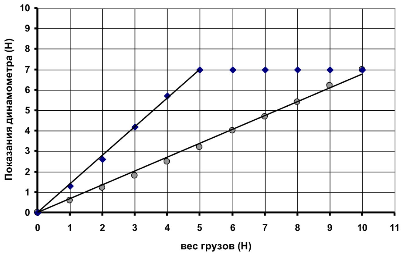
Зависимость показаний динамометра от веса грузов
