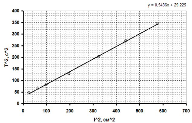
Рис.3 Зависимость квадрата периода от l^2
