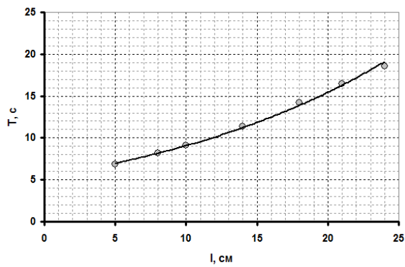
Рис.2 Зависимость периода от положения грузов
