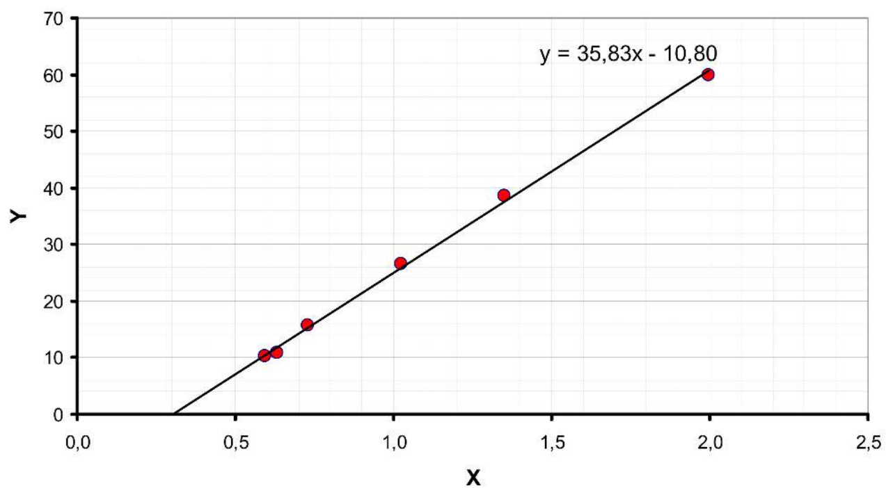
Соскальзывание (линеаризация)
