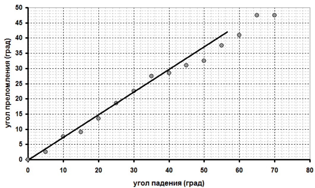
Рис. 2 Зависимость угла преломления от угла падения
