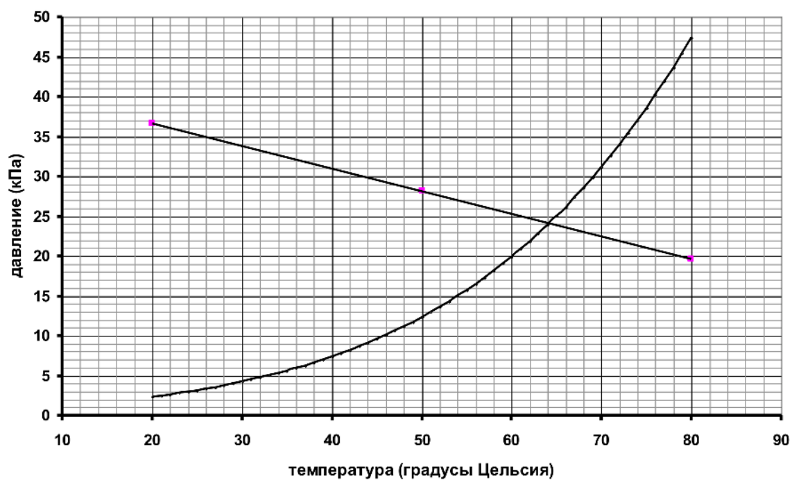
Зависимость давления насыщенных паров от температуры
