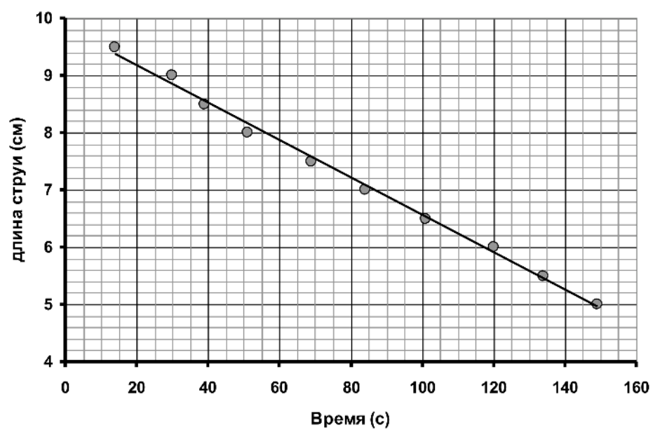
Зависимость длины струи от времени
