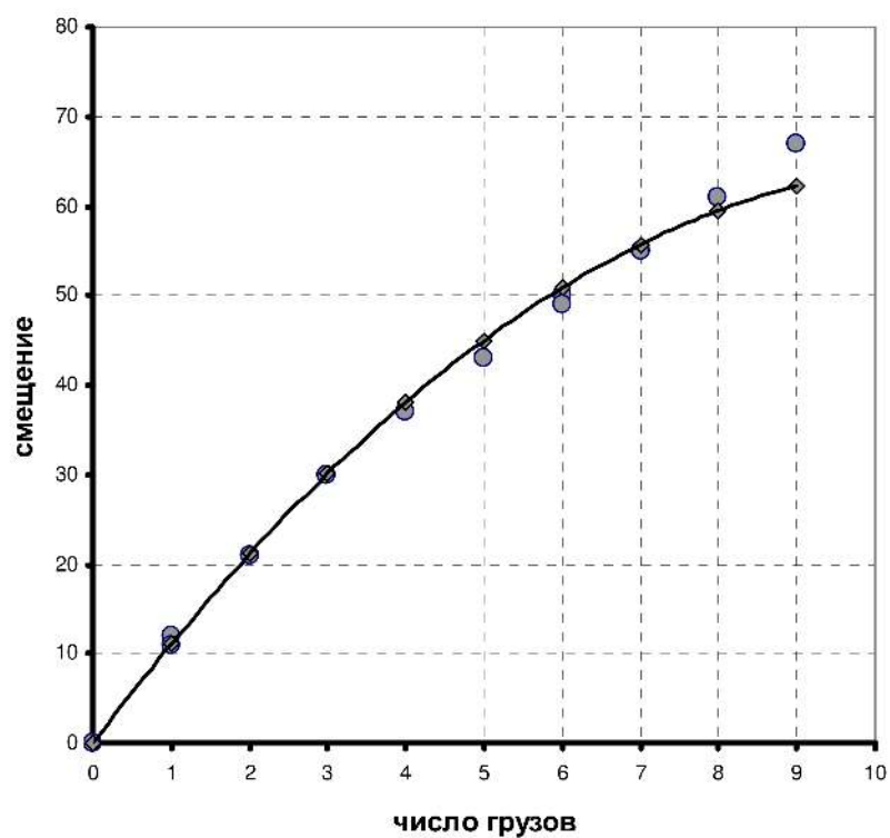
Вертикальное смещение "треугольной" пружины
