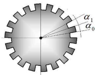
Колесо 1
