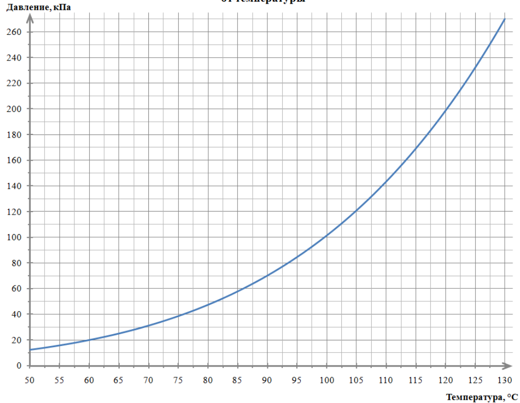
Зависимость давления насыщенного пара воды от температуры
