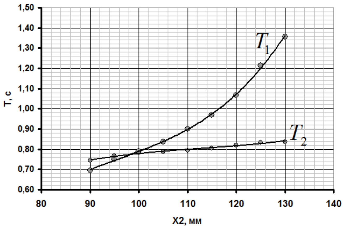
Зависимость периода колебаний от координаты
