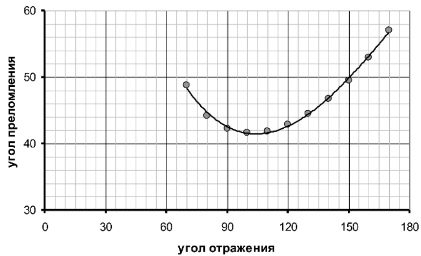
Преломление в призме
