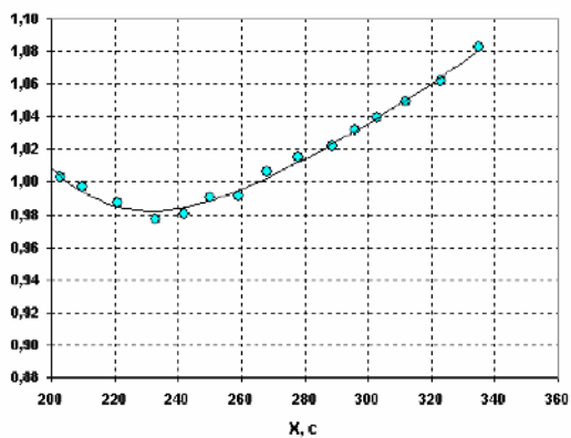
Период колебаний маятника с грузом
