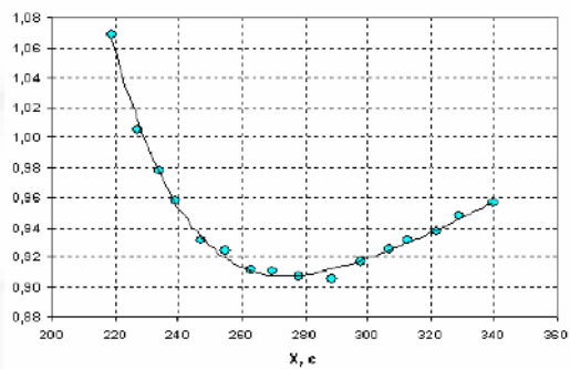
Период колебаний маятника без груза
