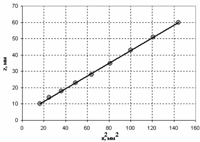
Зависимость смещения от точки подвеса (линеаризация)
