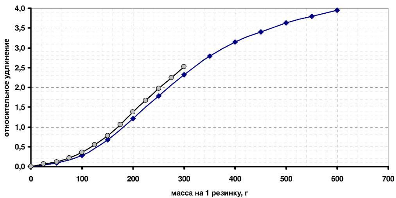
Рис. 2 Зависимость относительного удлинения от приведенной массы
