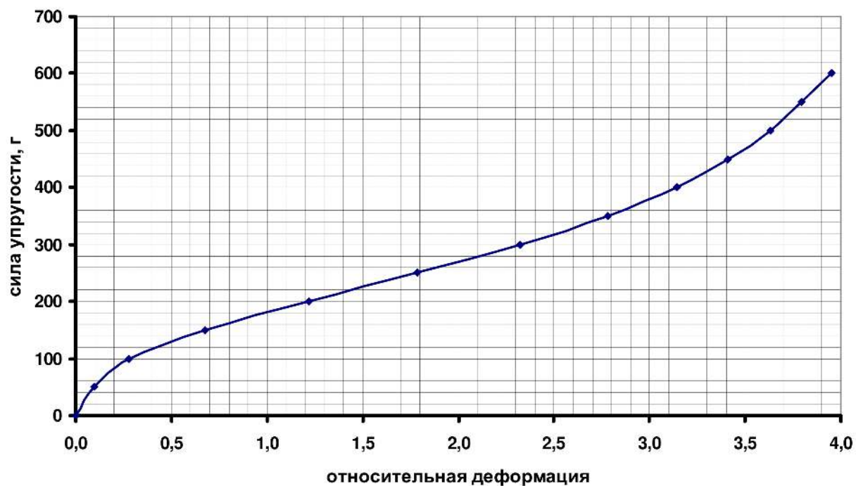
Рис. 4 Зависимость деформации резинки 2:3 от нагрузки
