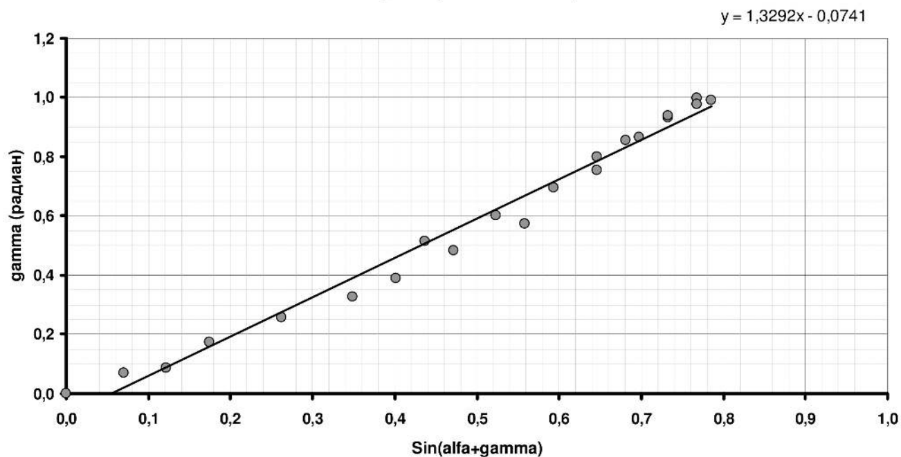
Рис. 2 Проверка закона Гука
