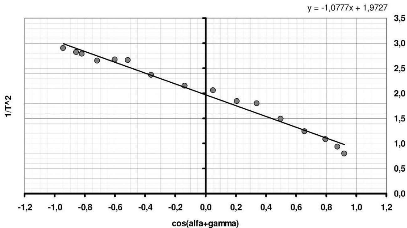
Рис. 3 Линеаризация формулы для периода
