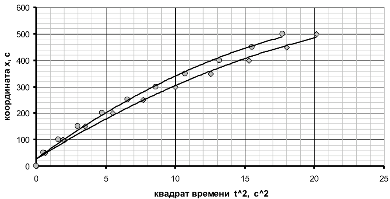
Закон движения трубки (неудачная попытка линеаризации)
