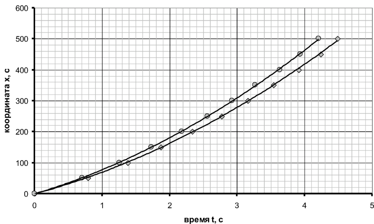
Закон движения трубки
