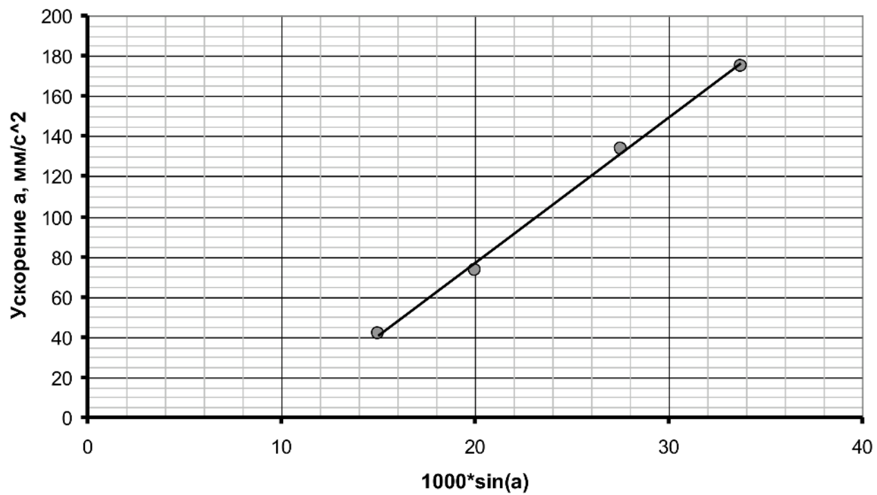
Зависимость ускорения от угла наклона
