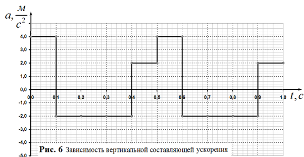
Рис. 6 Зависимость вертикальной составляющей ускорения центра масс человека от времени.
