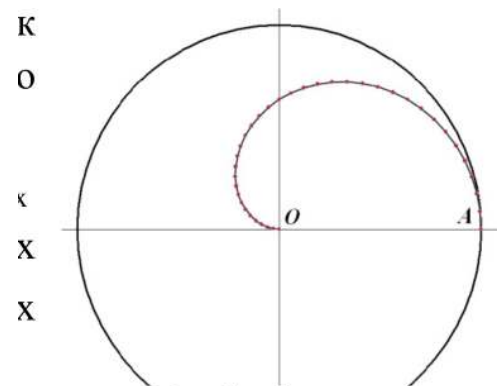
Рис. 7. Общий вид траектории центра масс при горении
