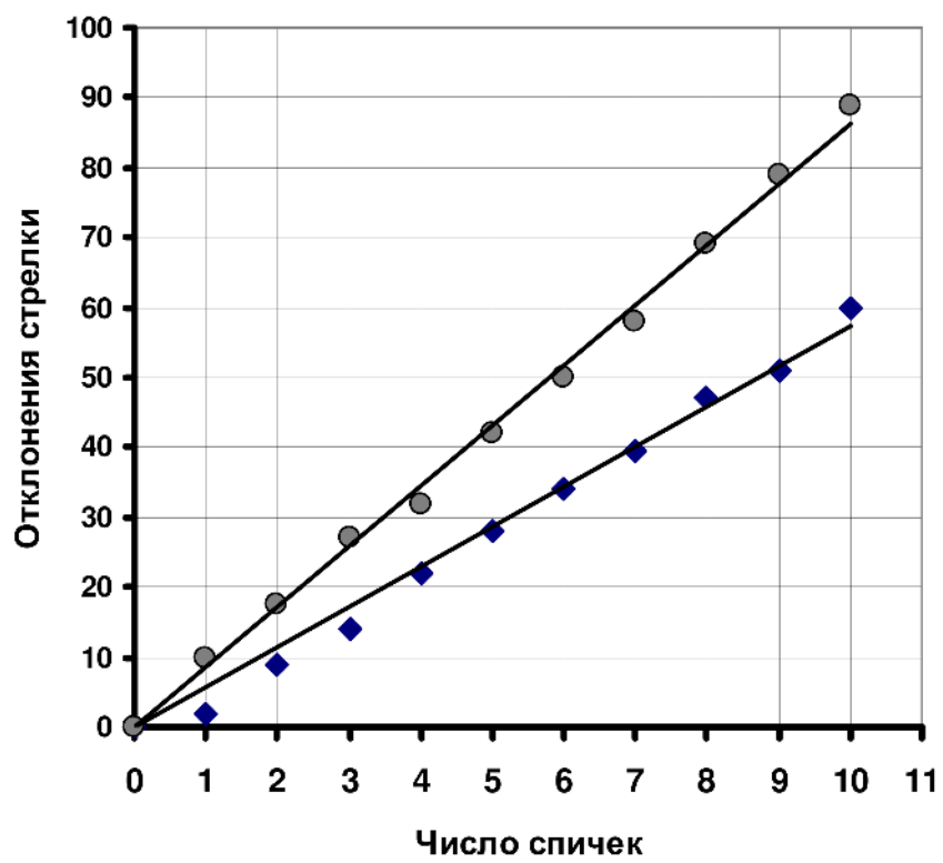
Градуировочные графики
