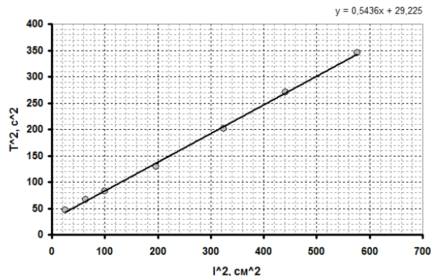
Рис.3 Зависимость квадрата периода от l^2
