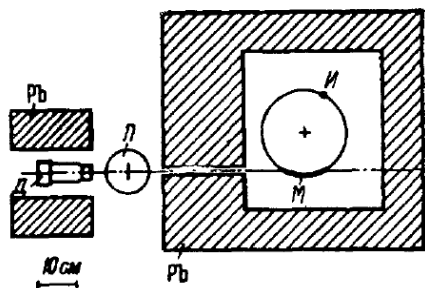
Рис. 2. Геометрия опыта. И — криостат с поглотителем ( T=88 K); М — вращающийся криостат с источником ( T=88 K); Д — детектор; И — источник.
